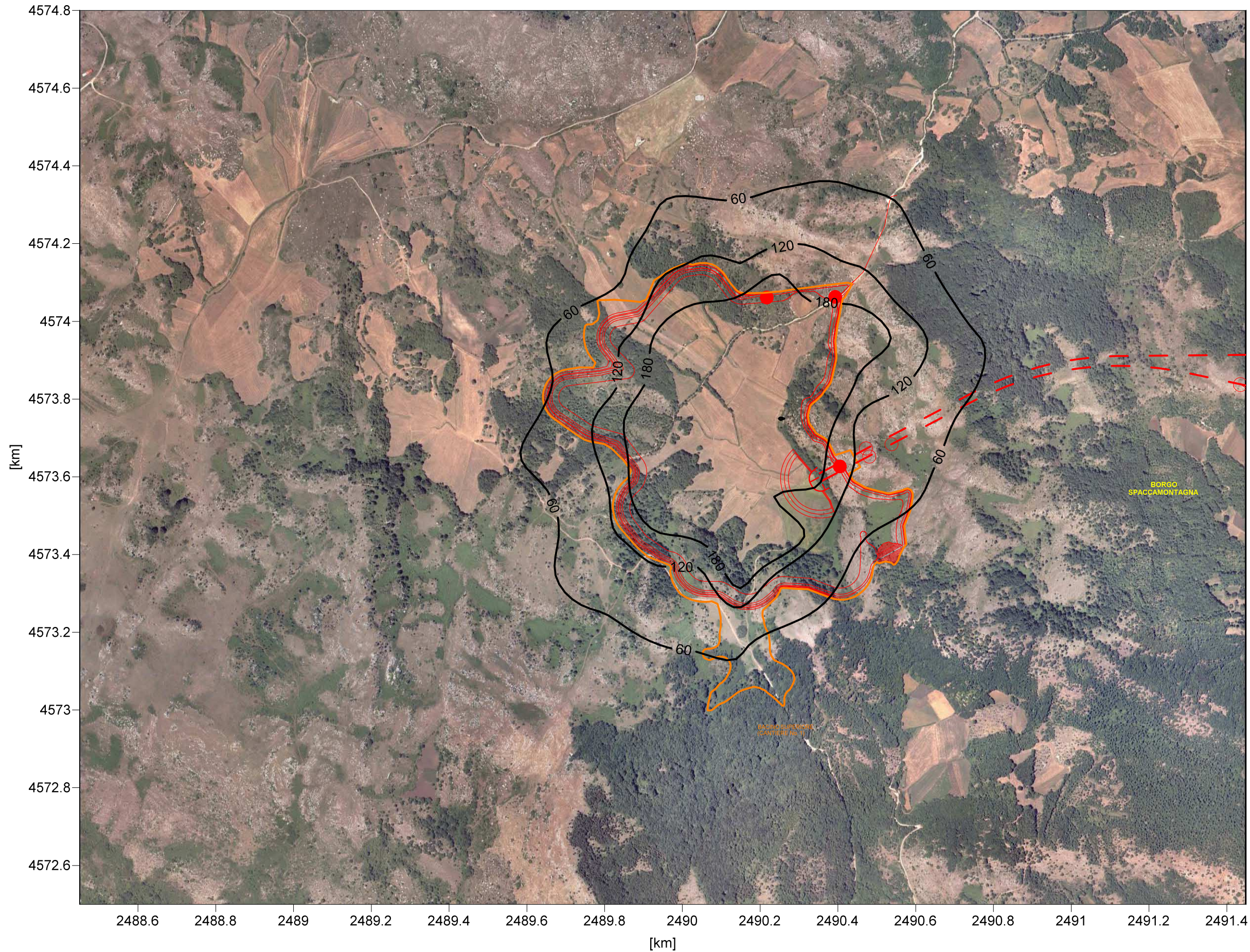
FIGURA 9.2 IMPIANTO DI REGOLAZIONE, CANTIERE No. 1, MAPPA DELLE RICADUTE AL SUOLO - NOx 99.8 PERCENTILE VALORE ORARIO
