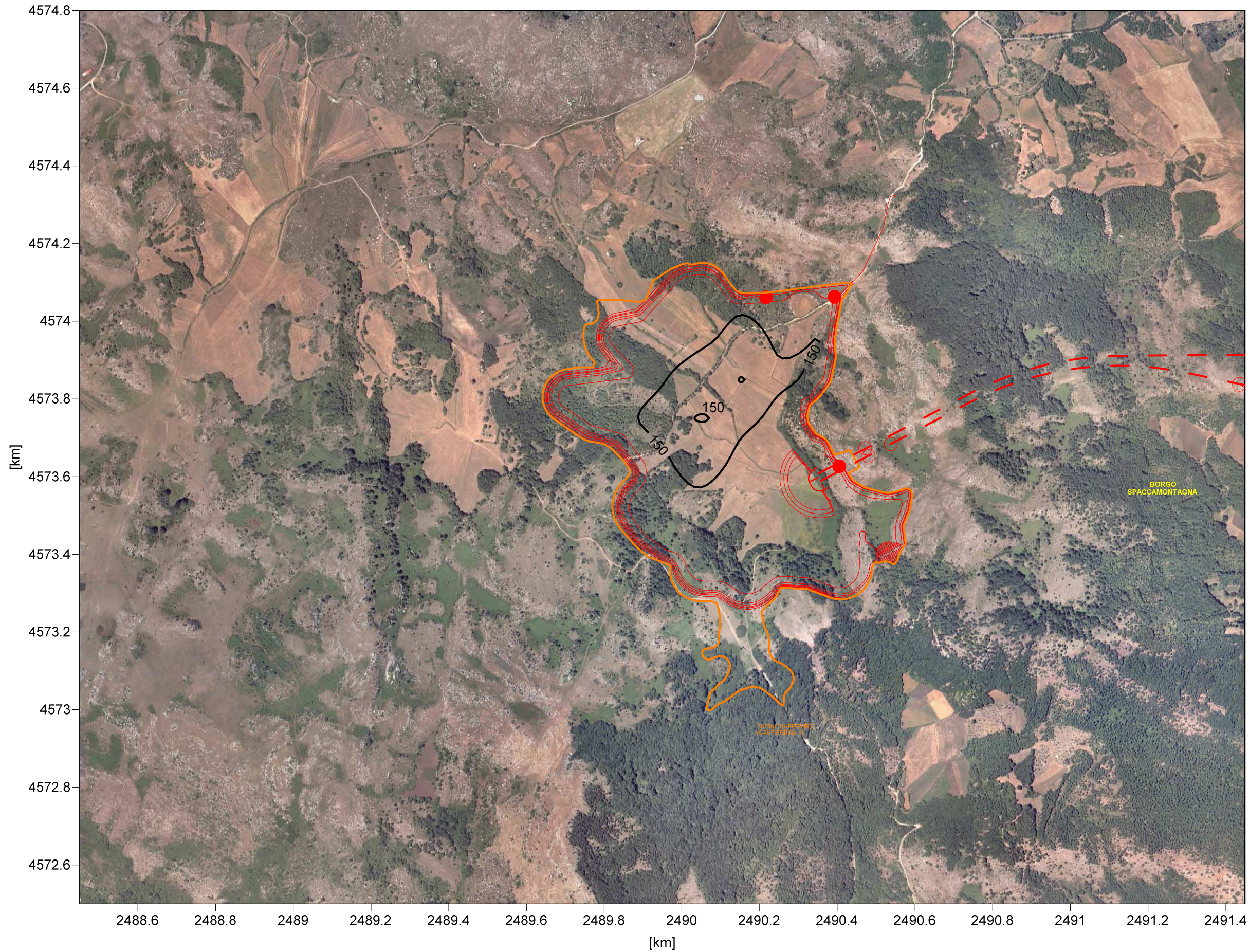
FIGURA 9.3 IMPIANTO DI REGOLAZIONE, CANTIERE No.1, MAPPA DELLE RICADUTE AL SUOLO - CO VALORE MEDIO MASSIMO GIORNALIERO CALCOLATO SU 8 H
