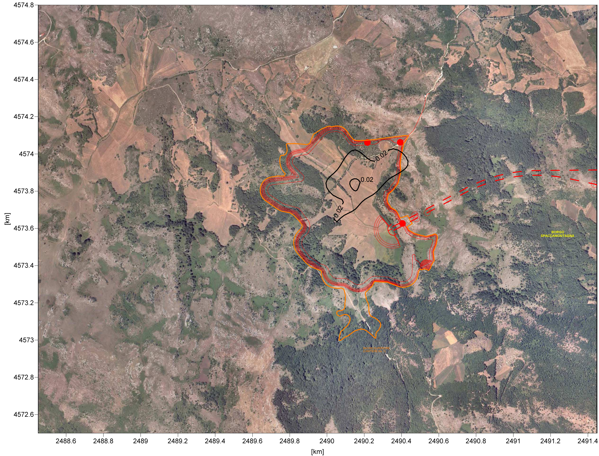
FIGURA 9.4 IMPIANTO DI REGOLAZIONE, CANTIERE No.1, MAPPA DELLE RICADUTE AL SUOLO - SOx VALORE MEDIO ANNUO
