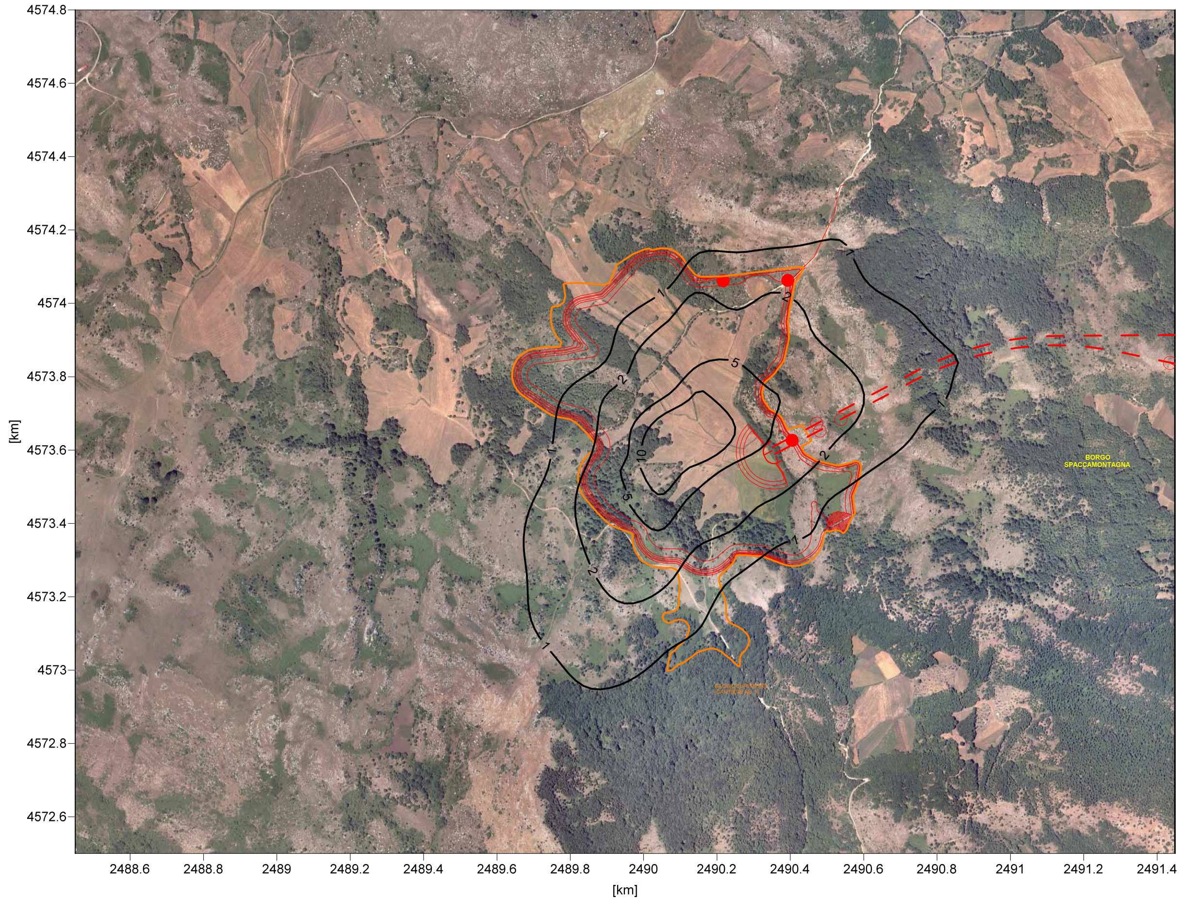
FIGURA 9.8 IMPIANTO DI REGOLAZIONE, CANTIERE No.1, MAPPA DELLE RICADUTE AL SUOLO - PM10 90.4 PERCENTILE VALORE GIORNALIERO
