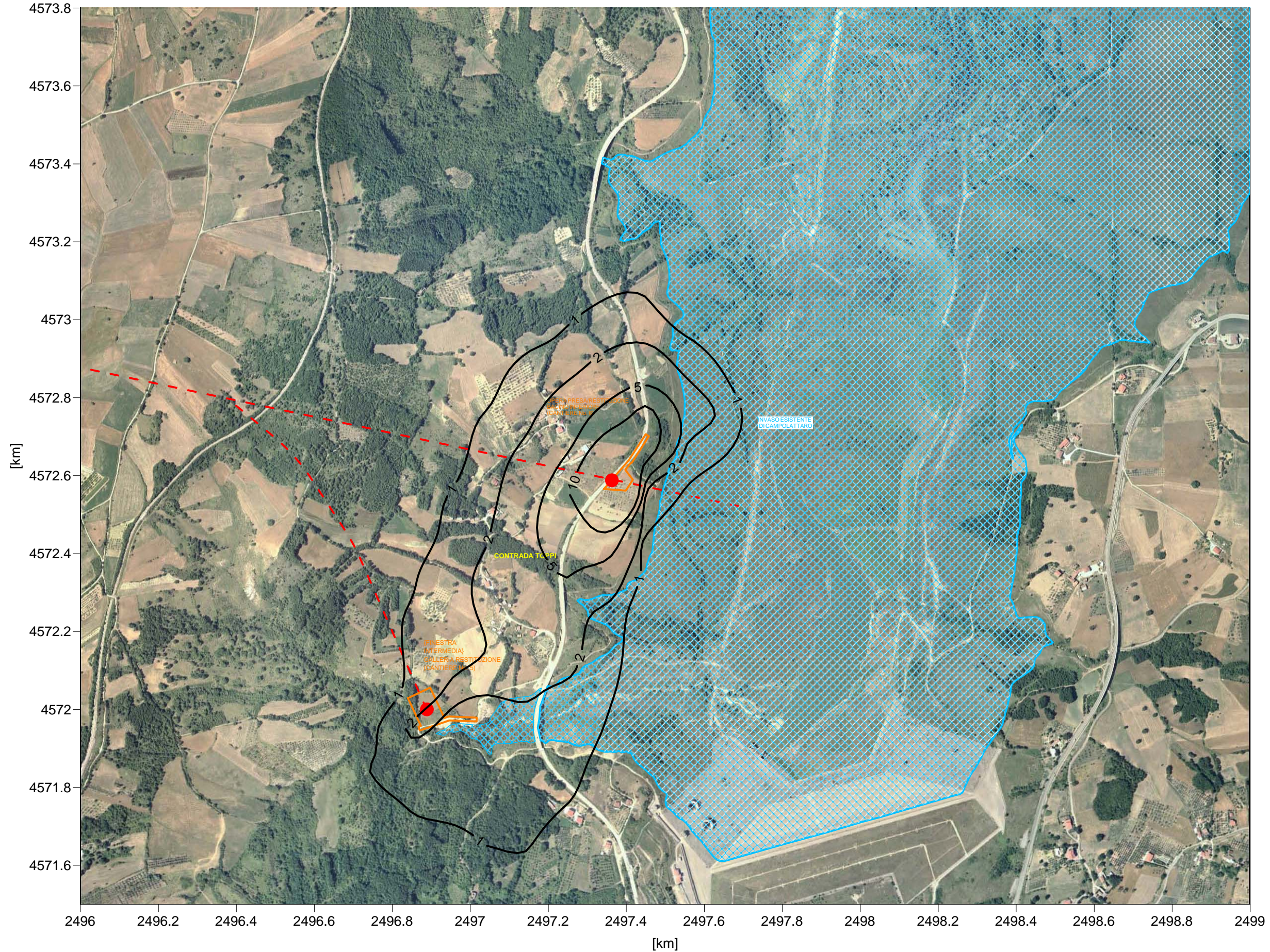
FIGURA 9.16 IMPIANTO DI REGOLAZIONE, CANTIERE No.5-6, MAPPA DELLE RICADUTE AL SUOLO - PM10 90.4 PERCENTILE VALORE GIORNALIERO
