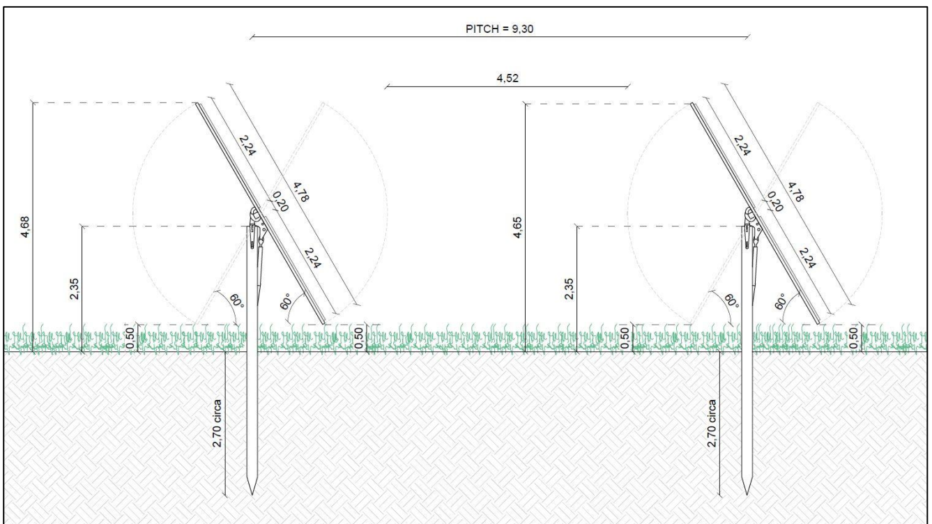
Particolare delle strutture di supporto dei moduli fotovoltaici
