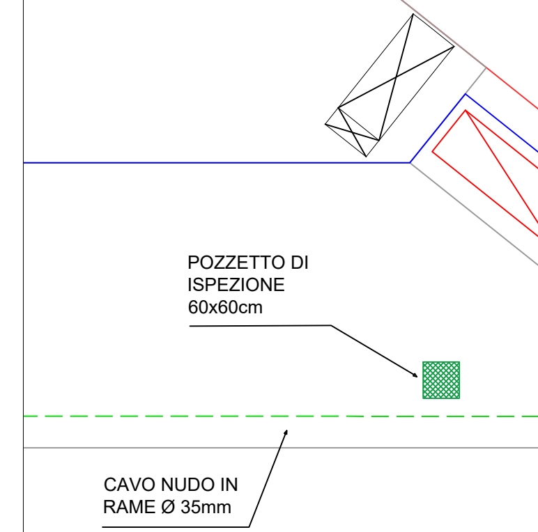
PARTICOLARE POZZETTO 2
