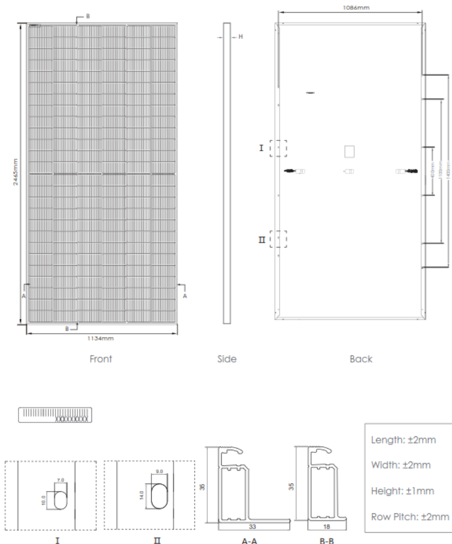
Figura 3.3 - Modulo fotovoltaico tipo: Inko solar 605Wp
