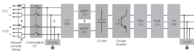
Figura 3.6 – Modulo inverter di stringa tipo SG250HX
