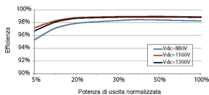
Figura 3.6 – Modulo inverter di stringa tipo SG250HX
