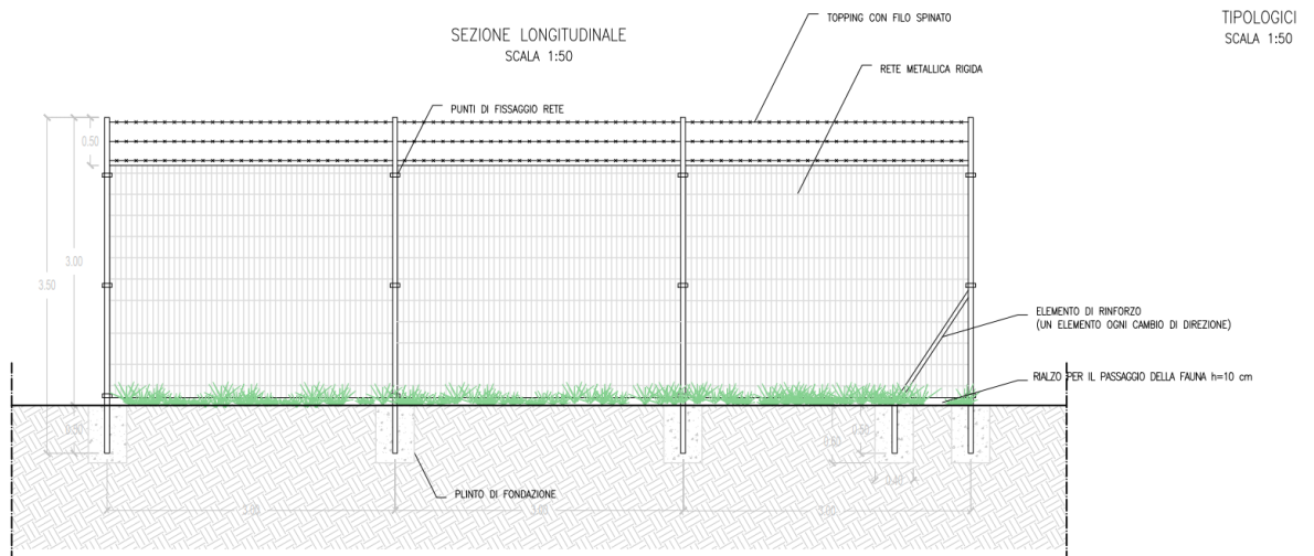
Figura 5.1: Tipico recinzione
