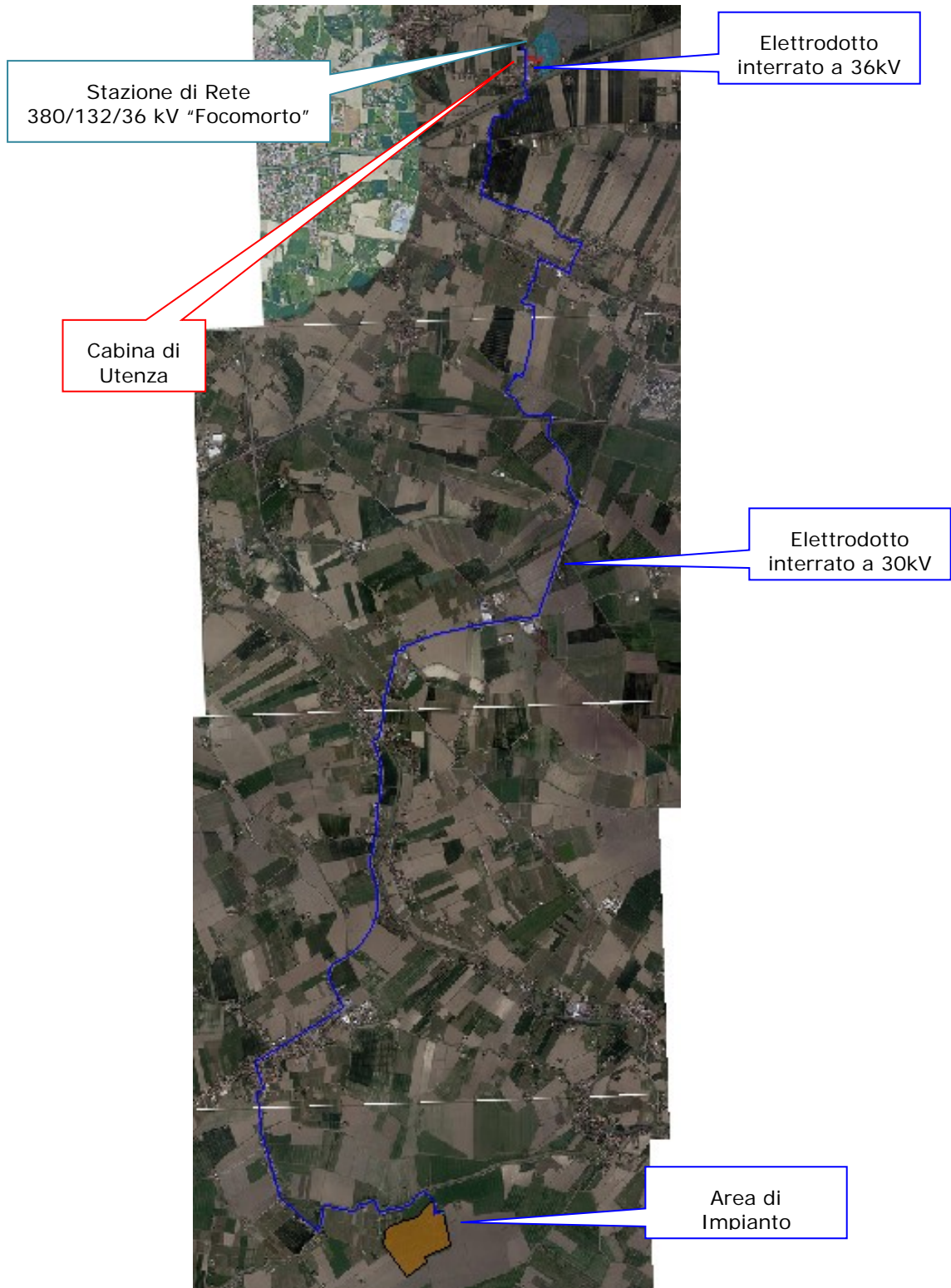
Figura 1: Tracciato degli elettrodotti MT e AT
