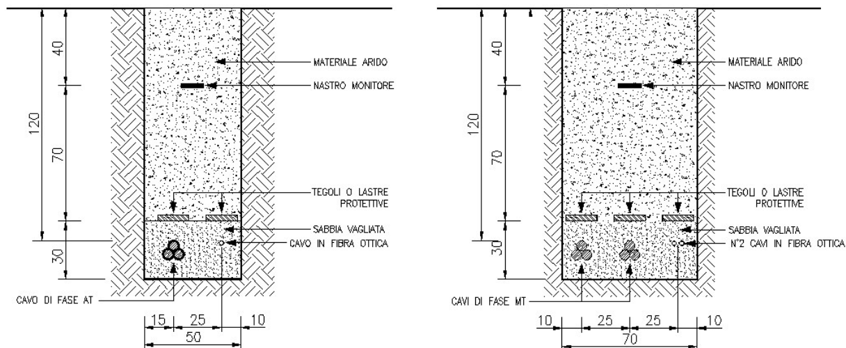
Figura 3: Tipici di posa cavi MT/AT con n°1 e 2 linee
