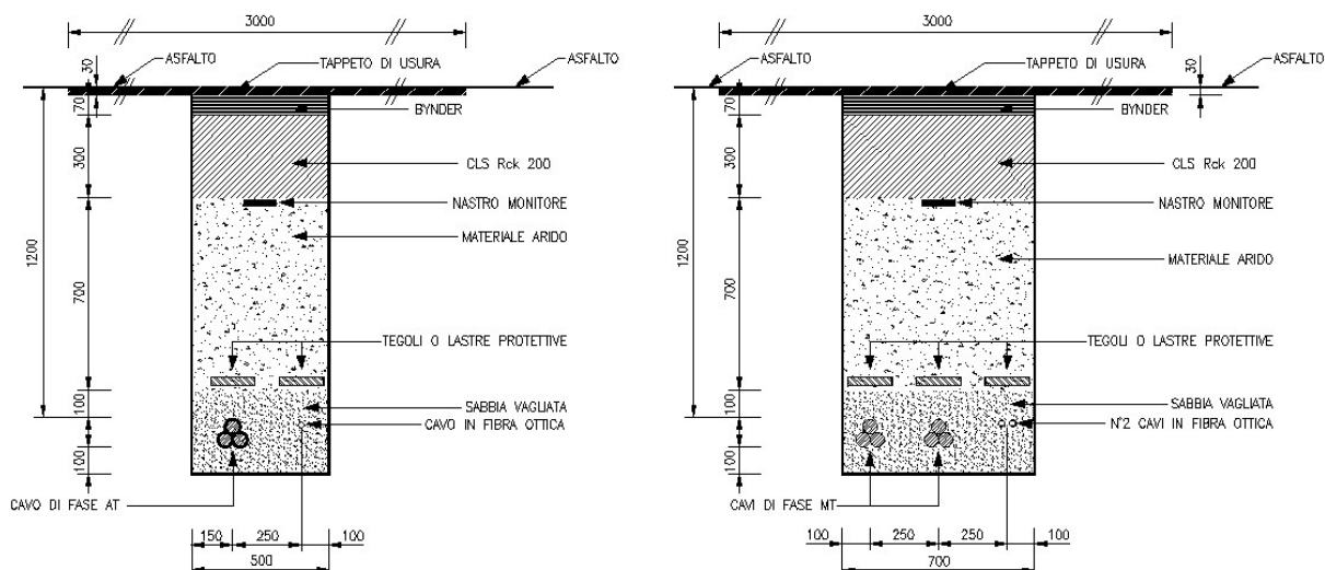
Figura 3: Tipici di posa cavi MT/AT con n°1 e 2 linee
