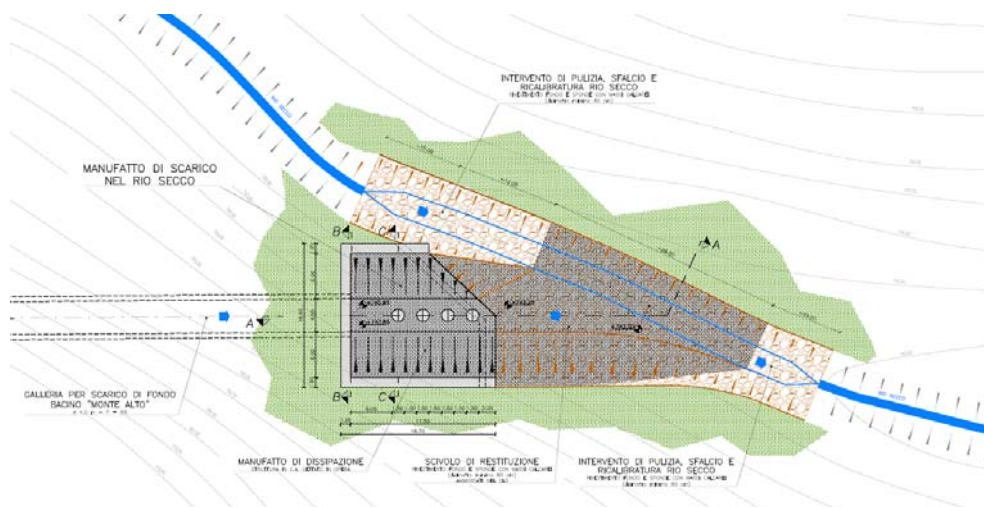
Figura 2.h: Manufatto di Dissipazione dello Sbocco dello Scarico di Fondo nel Rio Secco
