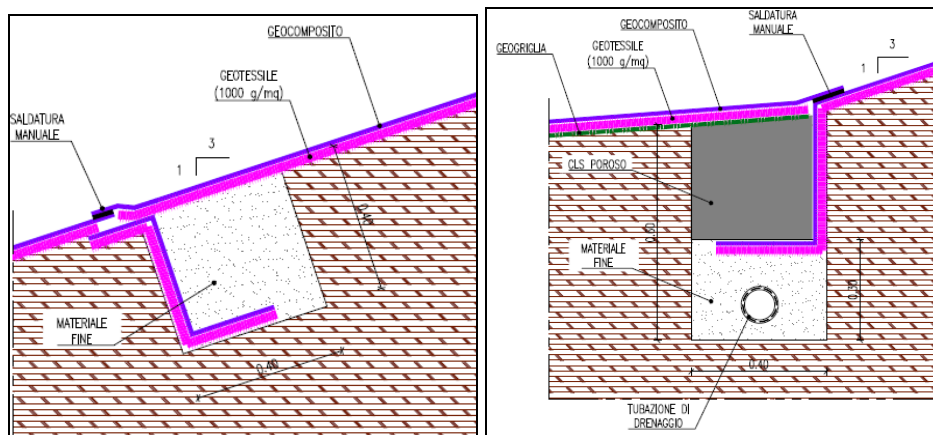
Figura 2.d: Collegamento Teli in PVC per Impermeabilizzazione Bacino di Monte Alto
