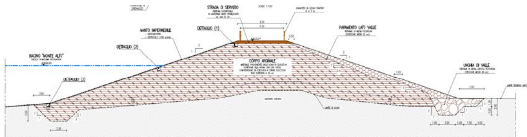
Figura 2.e: Sezione Tipo Argine Sud
