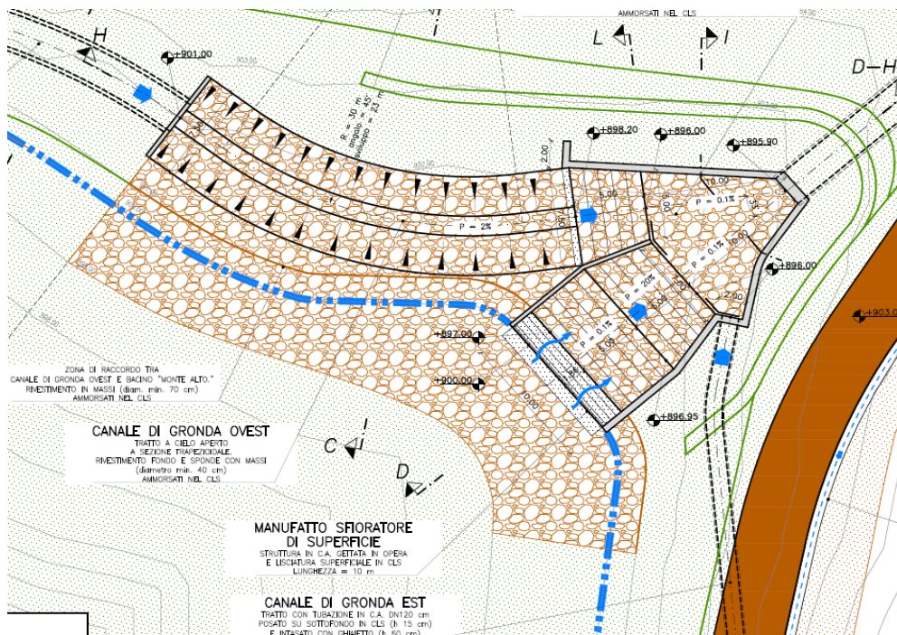
Figura 2.g: Pianta Manufatto di Confluenza
