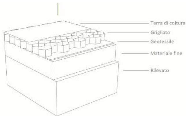
Figura 2.c: Sezione Tipologica Bordo Bacino
