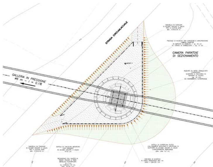
Figura 2.i: Stralcio Planimetrico Piazzale di Accesso al Pozzo Paratoie di Valle
