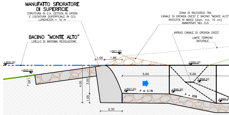
Figura 2.f: Sezione Manufatto Sfiatore di Superficie
