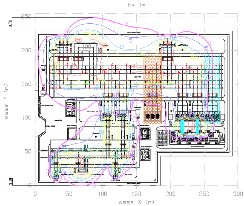
Calculations performed by software BE SHIELDING MAGIC Figura 7 – Livelli di campo magnetico a 1 m dal piano della stazione
