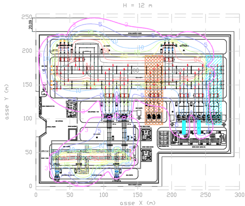
Calculations performed by software BE SHIELDING MAGIC Figura 10 – Livelli di campo magnetico a 12 m dal piano della stazione
