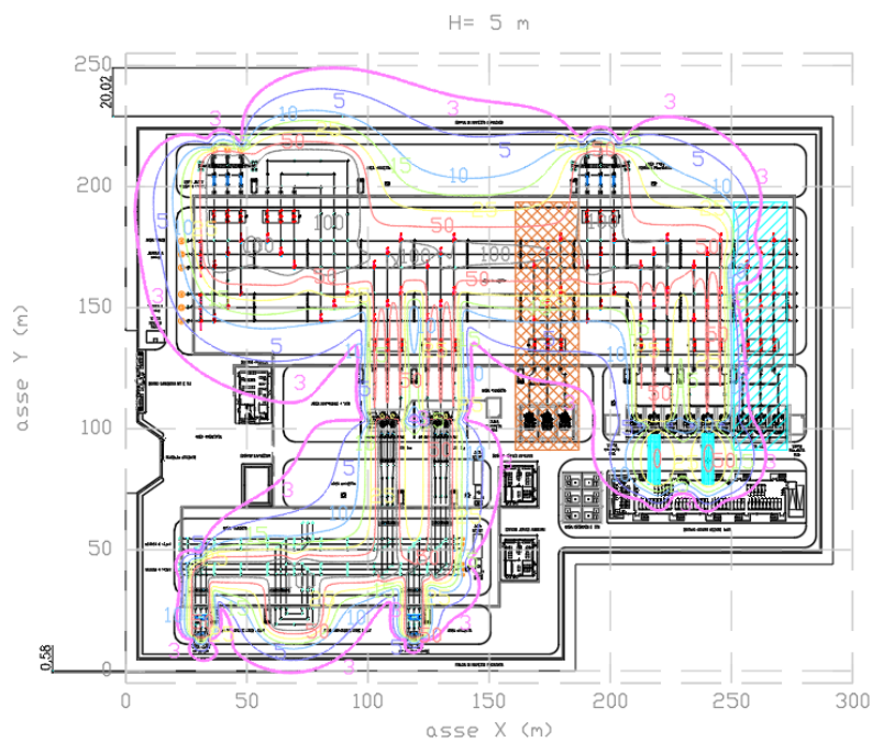
Calculations performed by software BE SHIELDING MAGIC Figura 8 – Livelli di campo magnetico a 5 m dal piano della stazione
