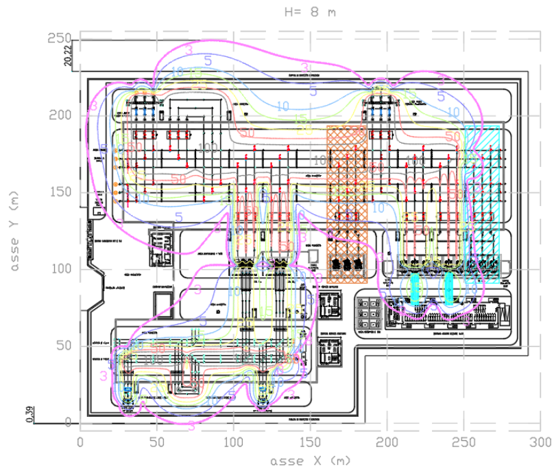
Calculations performed by software BE SHIELDING MAGIC Figura 9 – Livelli di campo magnetico a 8 m dal piano della stazione
