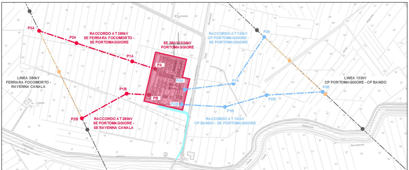
Figura 1: stralcio della planimetria con indicazione delle opere in progetto
