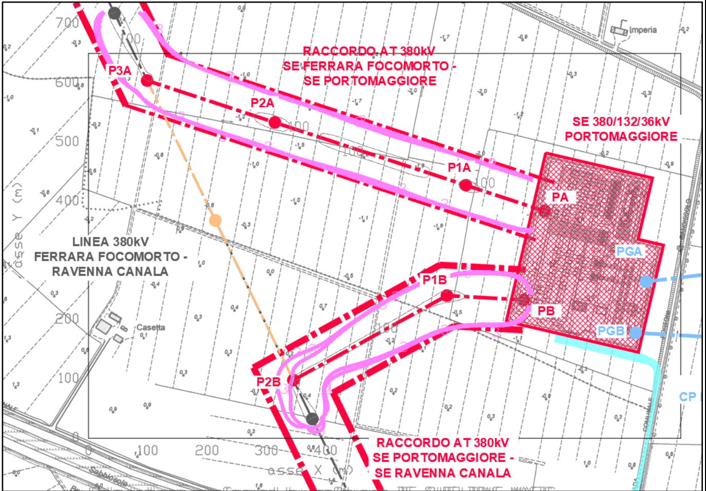
Figura 9 – Indicazione delle DPA e sintesi dei risultati delle simulazioni alle diverse altezze dal suolo
