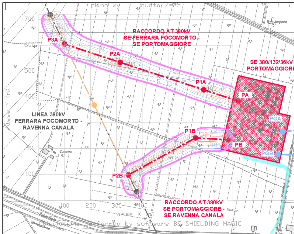
Figura 8 - Livello di campo magnetico generato dai raccordi a 25 mslm
