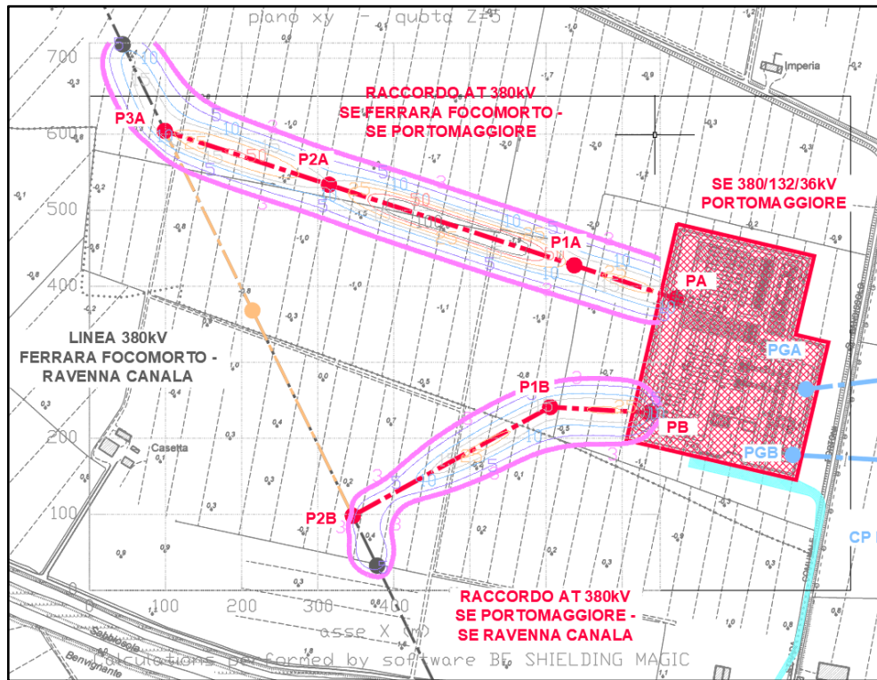
Figura 6 - Livello di campo magnetico generato dai raccordi a 5 mslm
