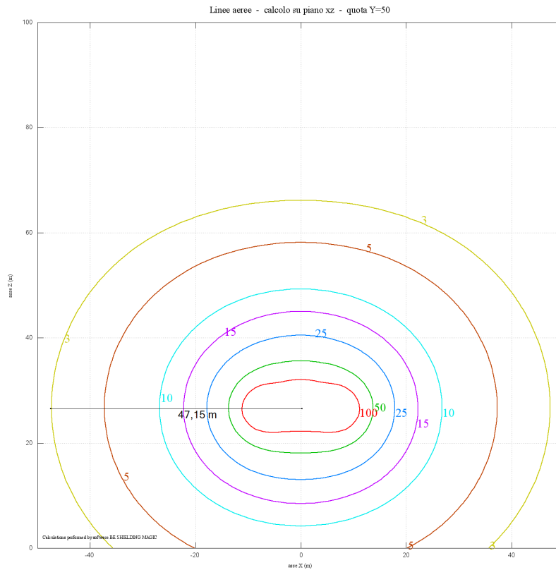
Figura 3 – Livelli di campo magnetico prodotti dalla configurazione dei conduttori su sostegno a Y in rettilo
