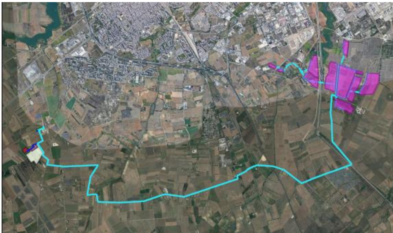
Figura 4-2 Percorso del Cavidotto interrato
