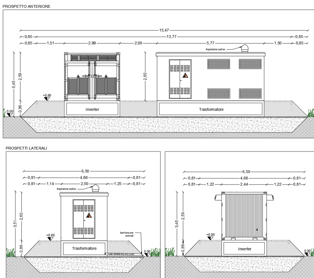
Figura 4-6 Cabine di campo
