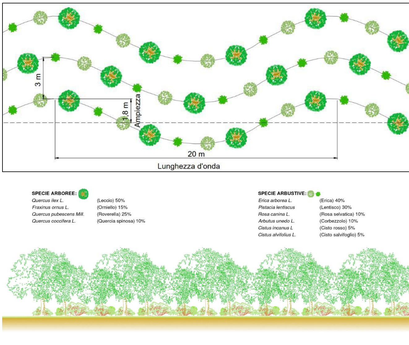
Figura 4-27: Schema di Impianto
