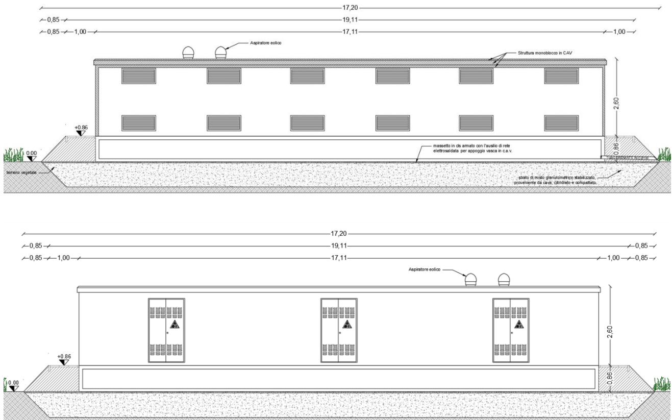
Figura 4-7 Cabine di raccolta
