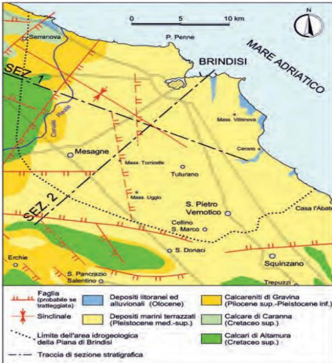
Figura 5-11: Carta geologico-strutturale della Piana di Brindisi (Fonte ISPRA)
