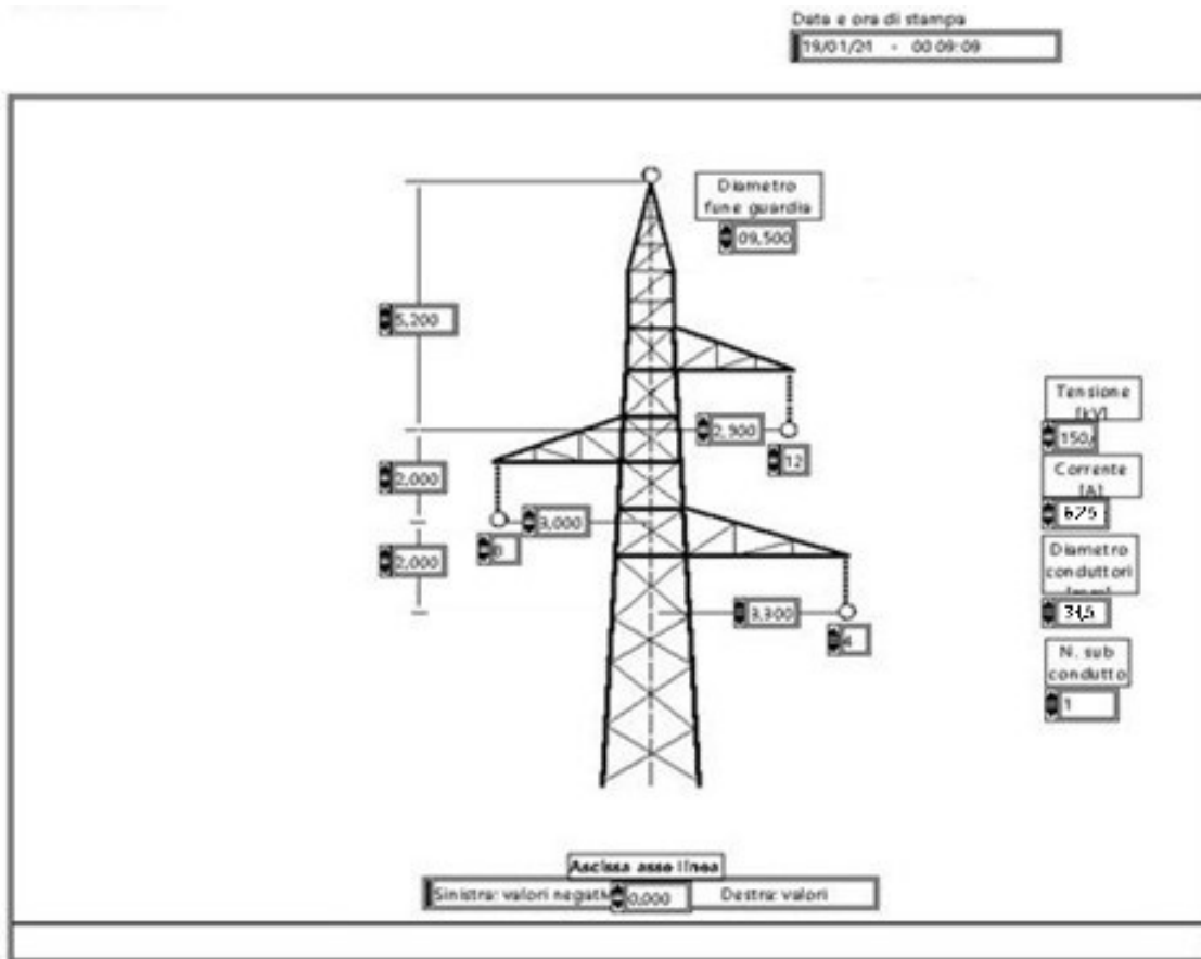
Figura 2: Geometria testa del sostegno in amarro con mensole disposte a triangolo.
