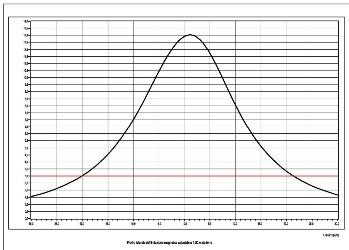
Figura 1: andamento dell'induzione magnetica in una sezione perpendicolare agli assi delle linea, calcolata ad 1,5 m dal suolo nel caso di franco minimo pari a 8,0 m per il sostegno di amarro con mensole a triangolo (in rosso l'obiettivo di qualità pari a 3 \mu T).
