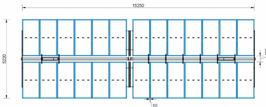
Figura 4-2 Tipologico struttura sostegno moduli - pianta
