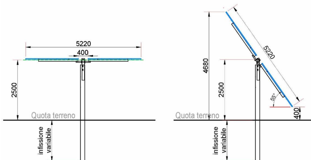
Figura 4-3 Viste laterali delle strutture di sostegno dei pannelli
