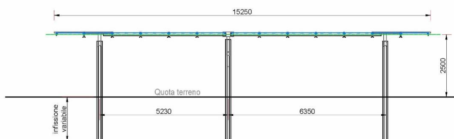
Figura 4-1 Tipologico struttura sostegno moduli – prospetto
