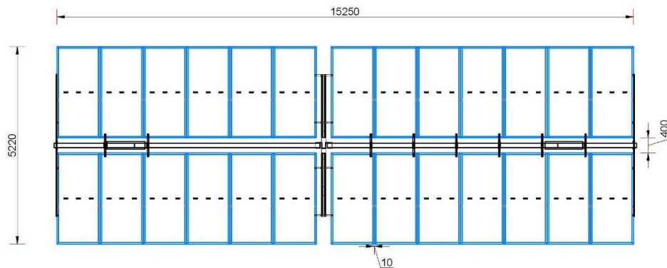
Figura 7 – Tipologico struttura sostegno moduli – pianta
