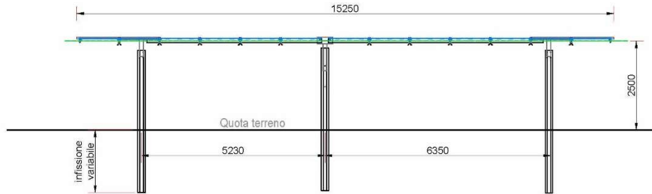
Figura 6 – Tipologico struttura sostegno moduli – prospetto
