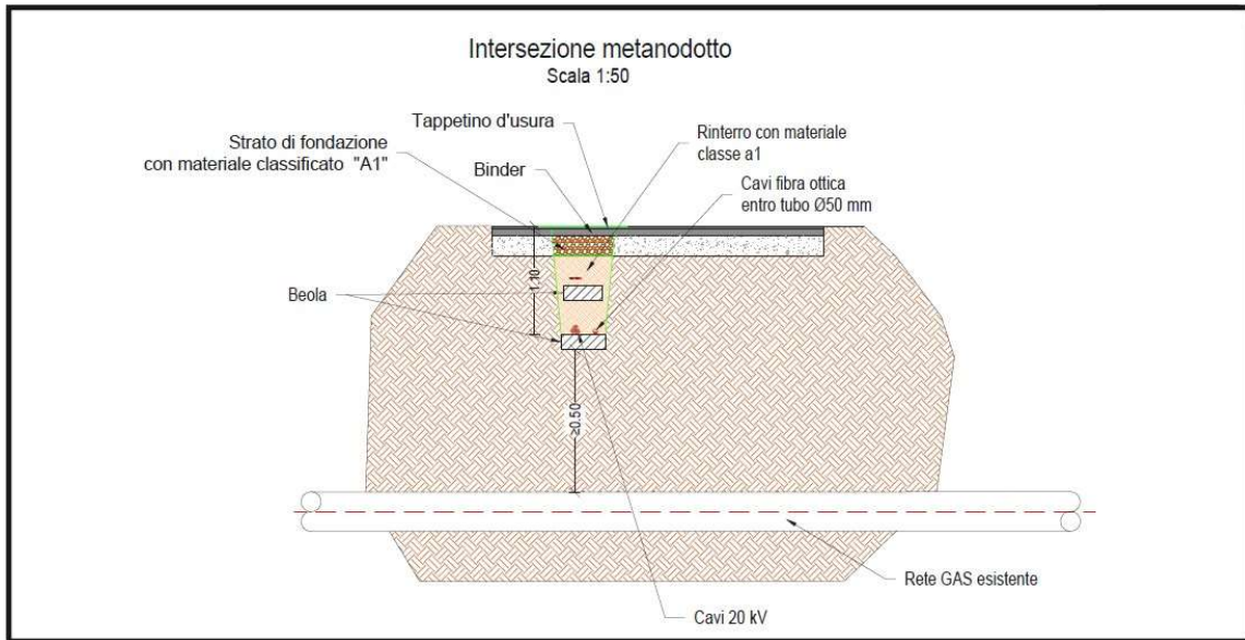
Figura 22 – Attraversamenti metanodotti
