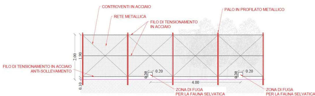
Figura 17 – Tipologico recinzione
