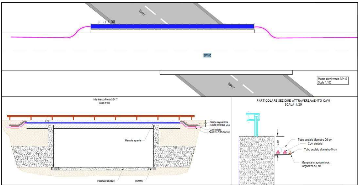
Figura 21 – Attraversamenti ponti
