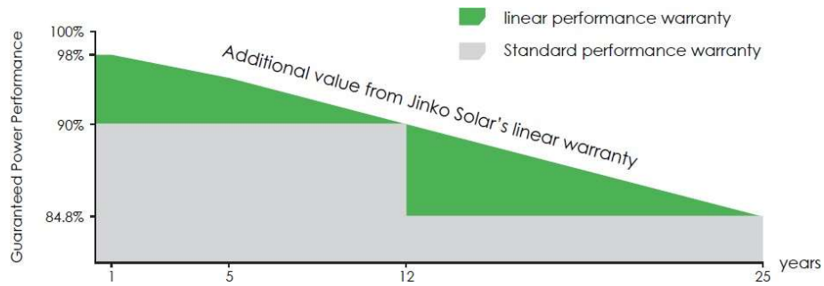
Figura 9 – Prestazioni garantite modulo fotovoltaico
