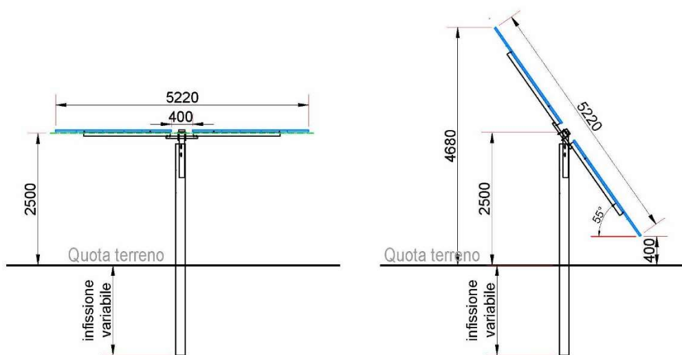
Figura 8 – Viste laterali delle strutture di sostegno dei pannelli
