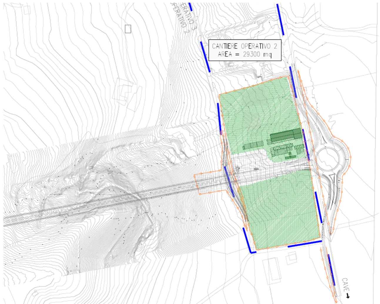
Figura 1-17 Cantiere operativo 2
