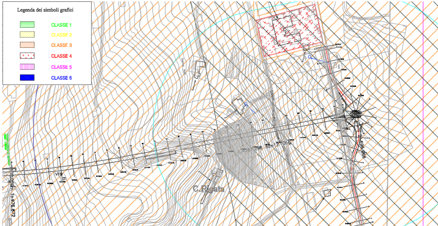
Figura 1-13 Zonizzazione acustica innesto Ovest della nuova tangenziale
