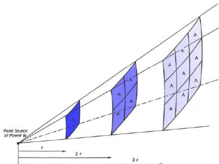
Figura 1-2 Fenomeno della divergenza nei fenomeni ondulatori. Definendo W la potenza sonora alla sorgente, l'intensità I dell'energia sonora è data da:
