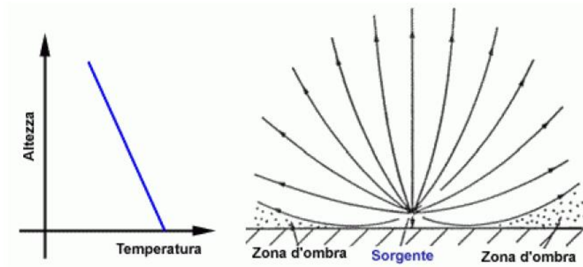
Figura 1-4 Effetto della temperatura con gradiente normale.
