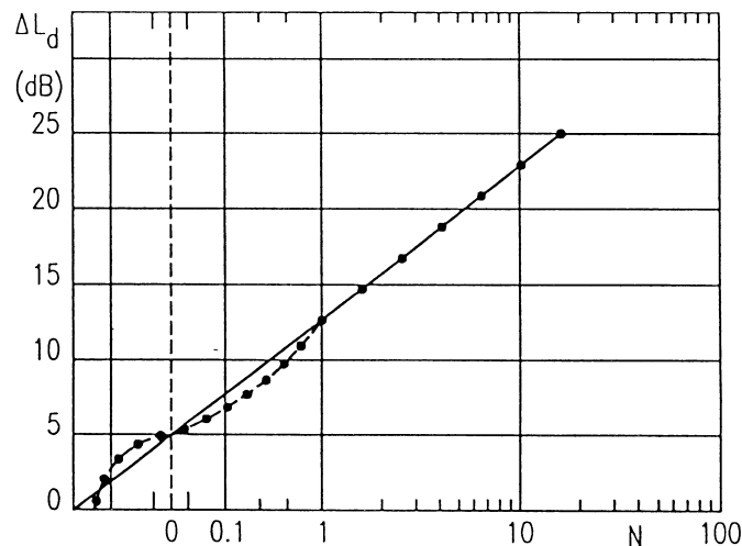
Figura 1-6 Diagramma di Maekawa per sorgenti lineari.
