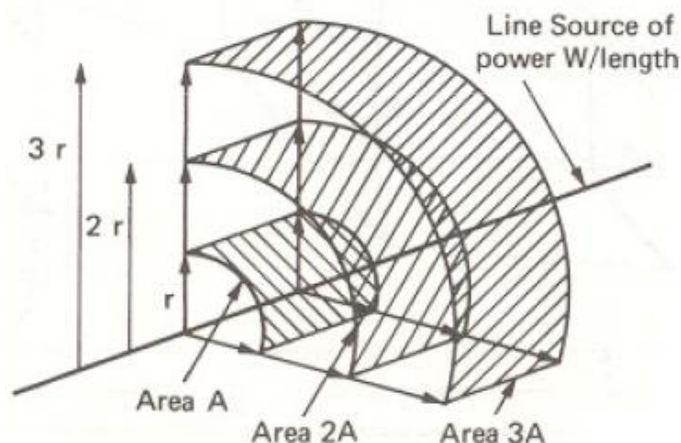
Figura 1-8 Propagazione delle onde sonore per sorgenti lineari.
