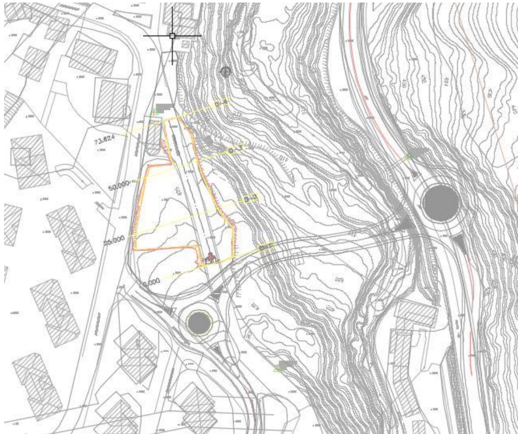
Figura 1-18 Cantiere operativo 3
