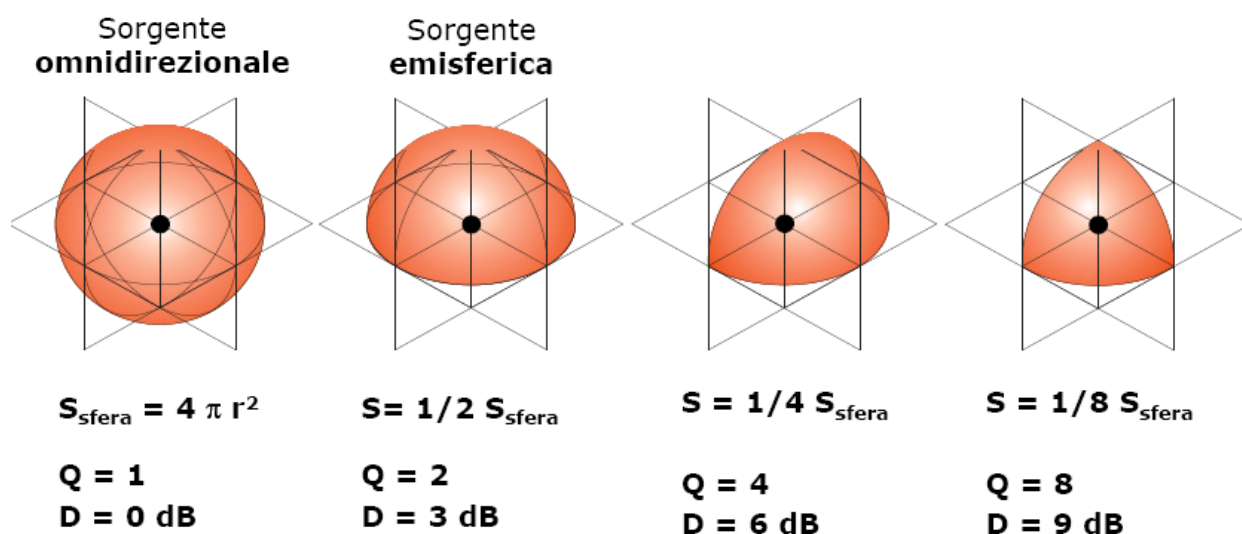
Figura 1-3 Fattori ed indici di direttività.
