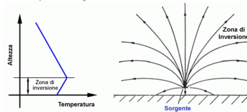
Figura 1-5 Effetto della temperatura in caso di inversione termica.
