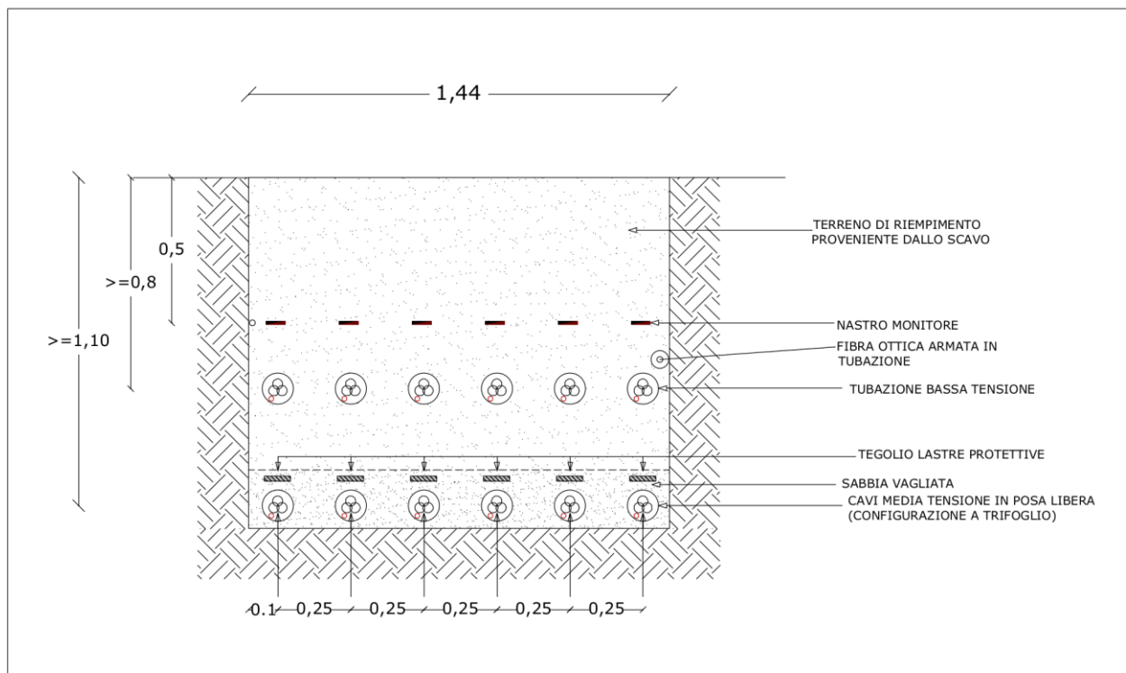
Figura: Sezione del cavidotto MT interno al campo "Baroninuovi".
