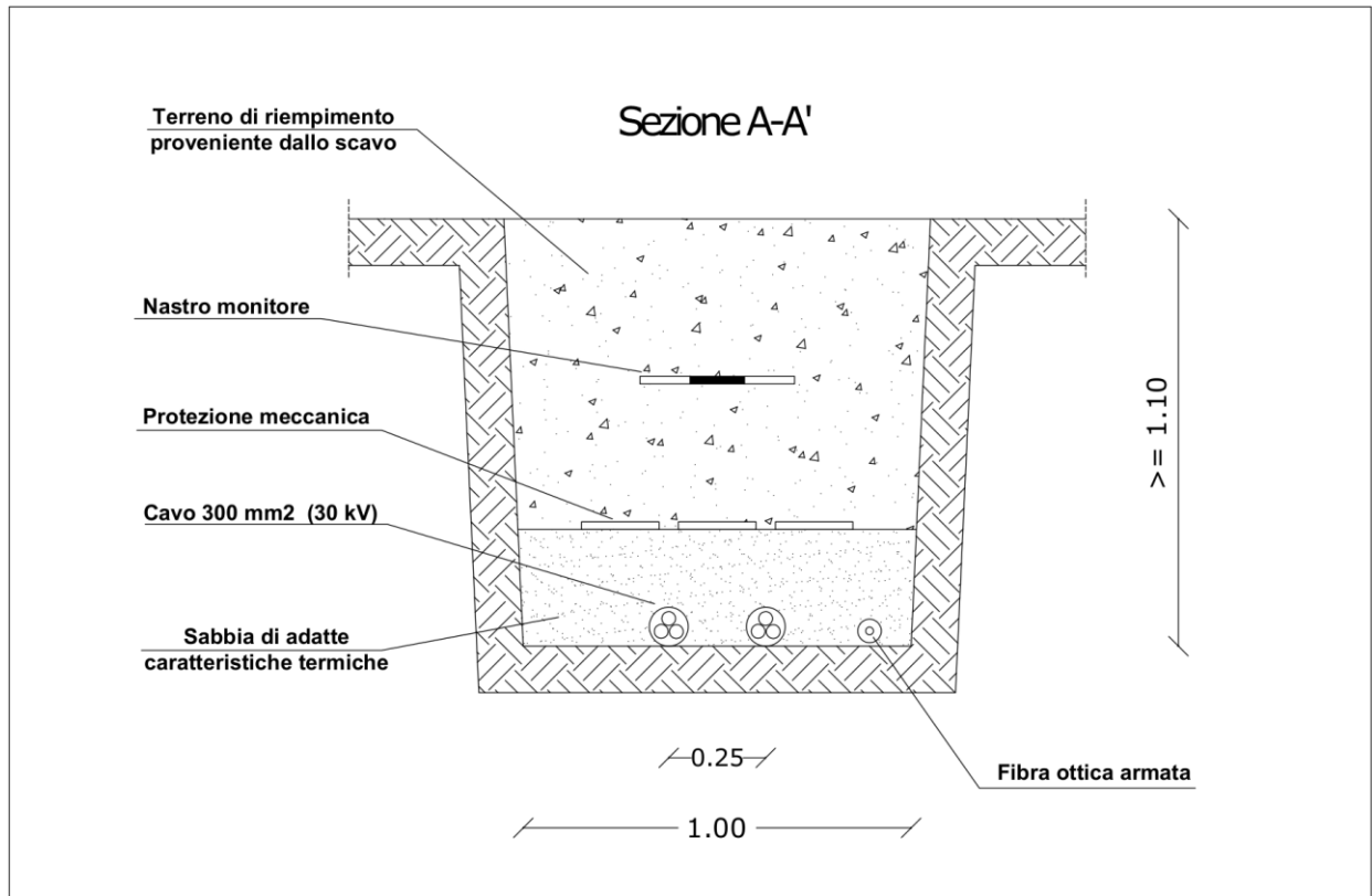
Figura: Sezione attinente all'interramento di cavi isolati in tubazioni in ingresso alla cabina di impianto.
