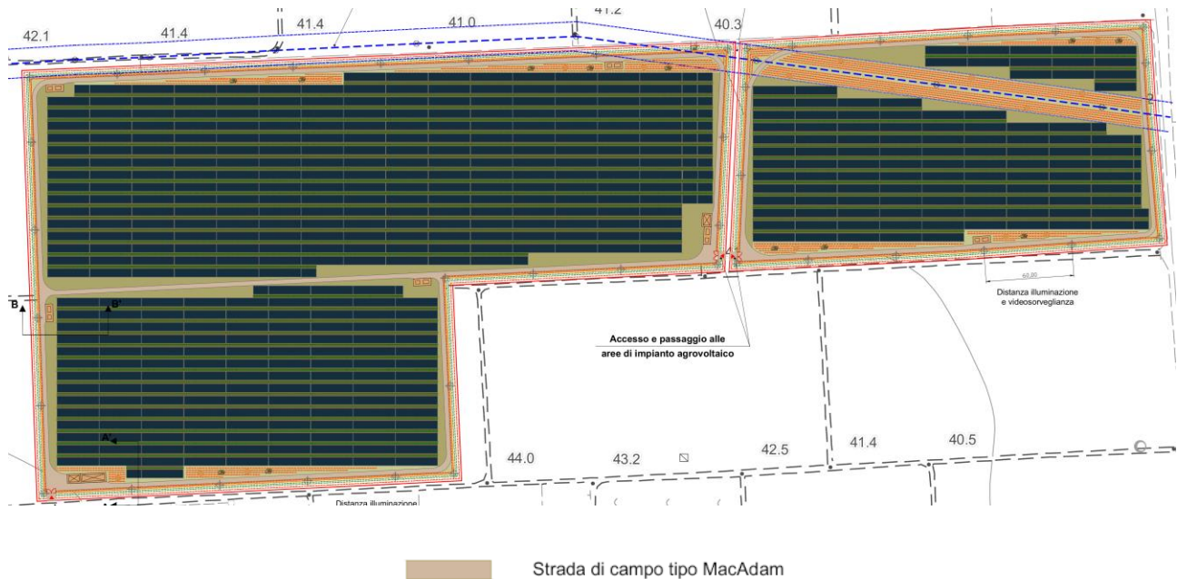
Figura: Layout di progetto con indicazione delle vie di servizio (strade di campo).
