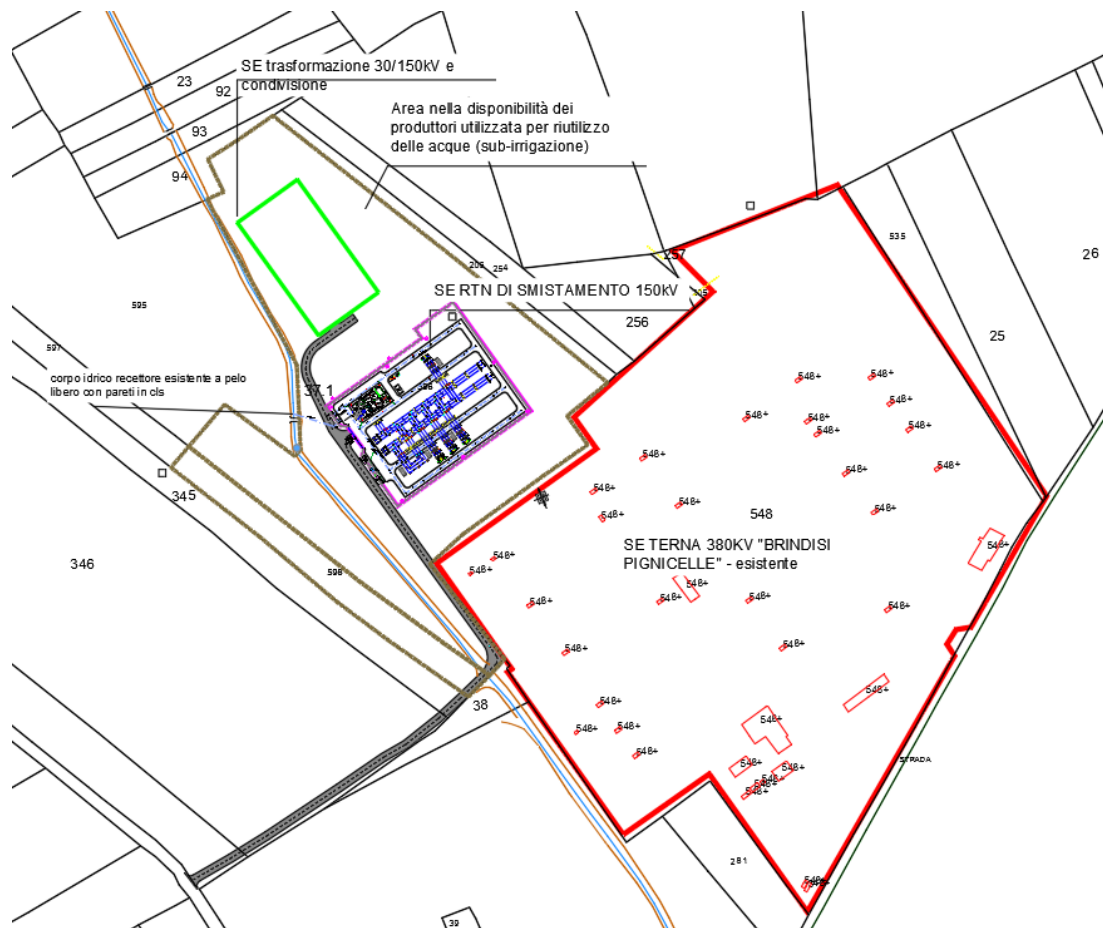
Figura 5: Inquadramento catastale dell'area destinata alla stazione utenza e stazione di smistamento
