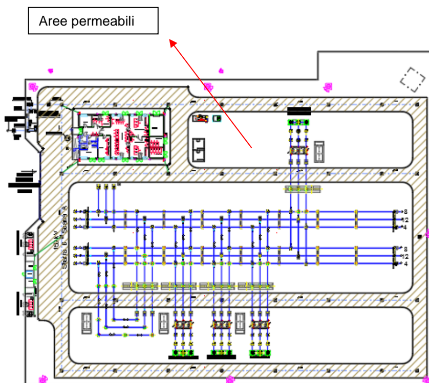
Figura 2: Le aree tratteggiate sono escluse dal calcolo delle portate poiché aree sterrate o con pietrisco.
