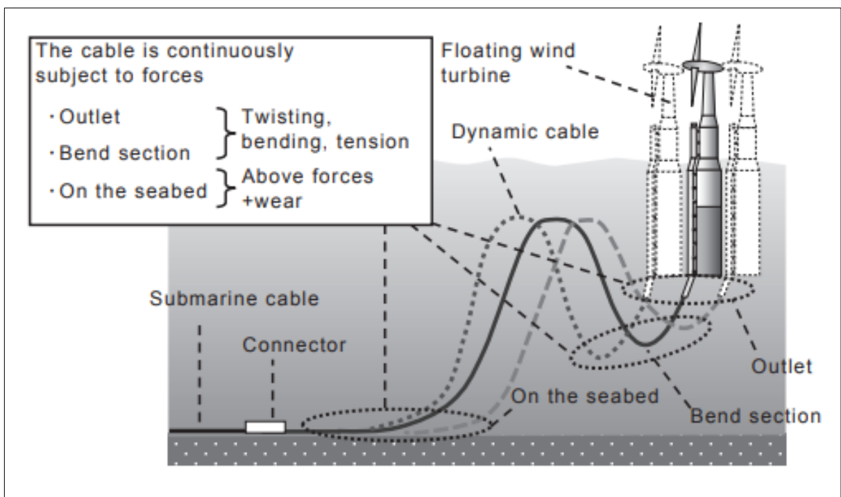
Figura 5.1: Collegamento via cavo a un impianto galleggiante di generazione di energia eolica offshore
