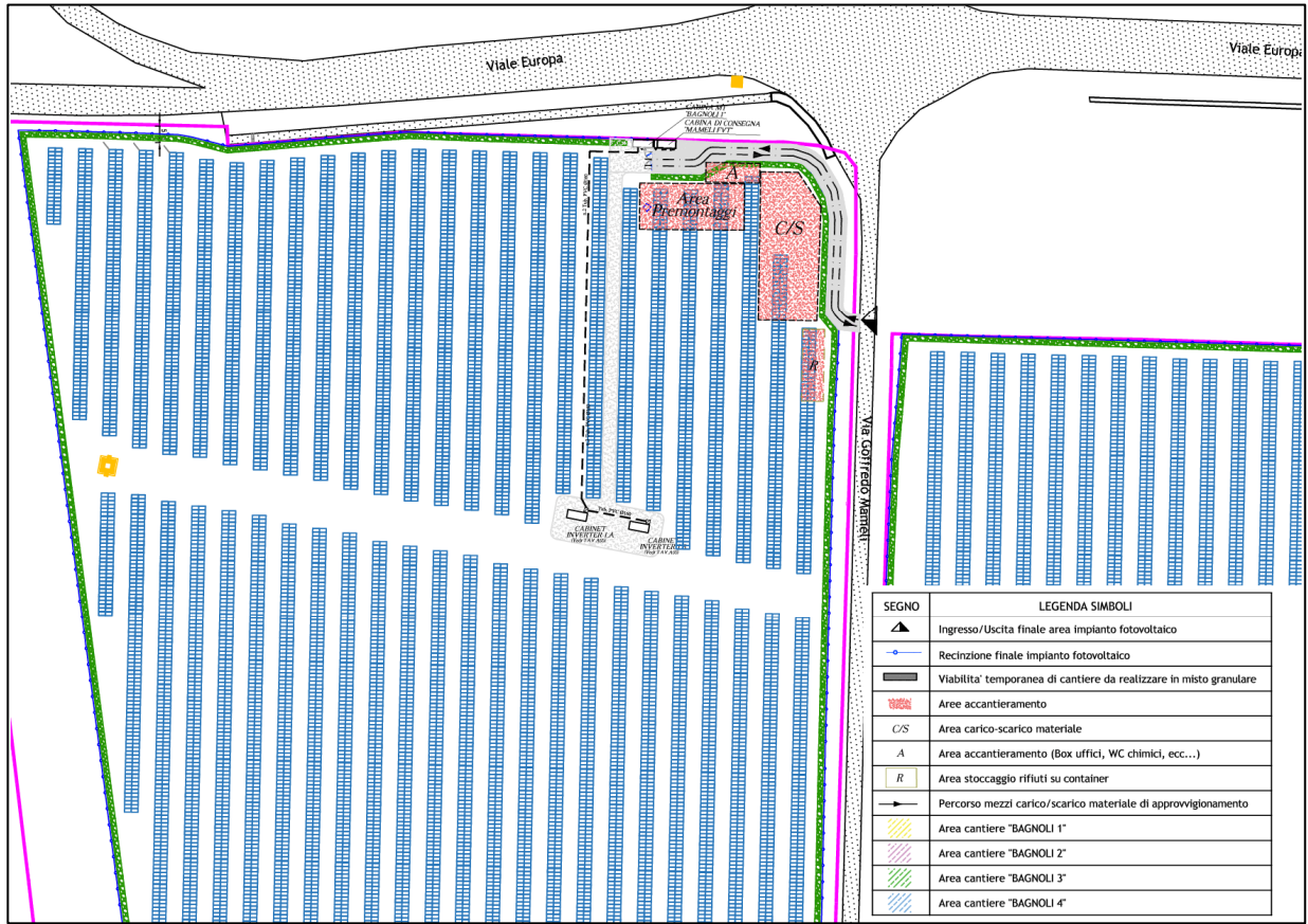
Figura 8 - Aree di cantiere impianto "BAGNOLI 1"
