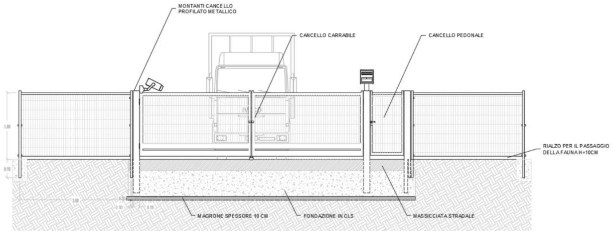
Figura 4.9 - Posizionamento sistema video sorveglianza e illuminazione esterna cancelli
