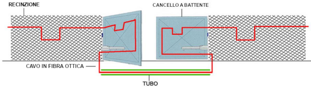
Figura 4.12 - Schema di installazione cavo in fibra ottica su recinzione.
