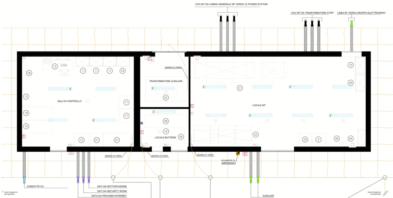
Figura 4.4 - Posizionamento plafoniere Cabina Generale MT.
