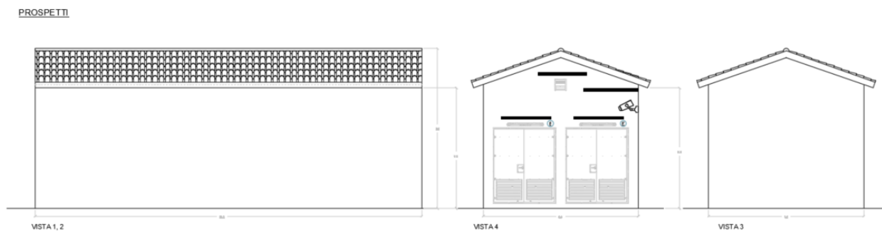
Figura 4.11 - 1151 Posizionamento sistema video sorveglianza e illuminazione esterna Magazzino
