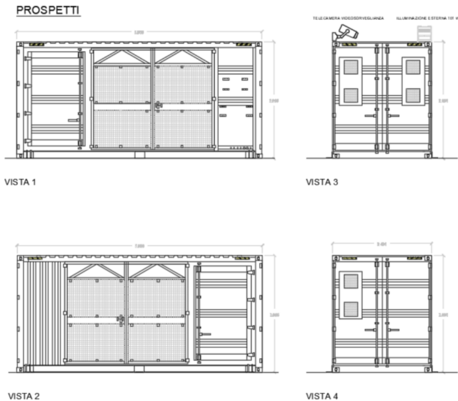
Figura 4.7 – Posizionamento sistema video sorveglianza e illuminazione esterna Power Station
