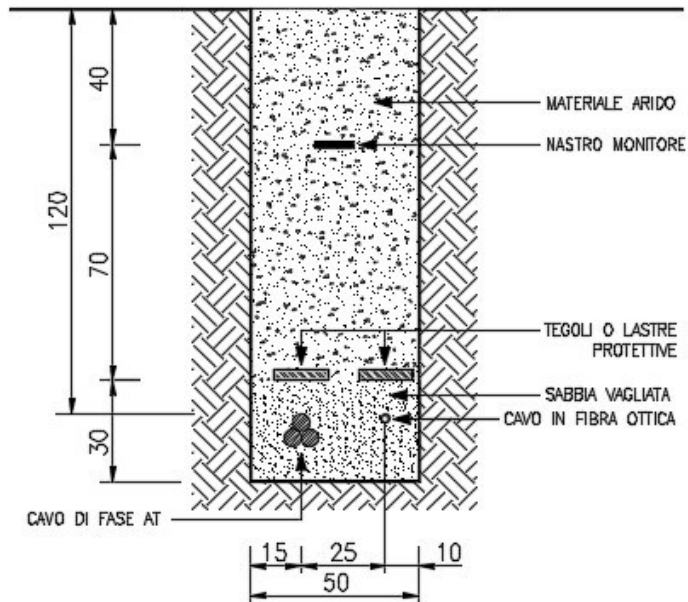
Figura 4: Tipici di posa cavo AT con n°1 linea su viabilità sterrata
