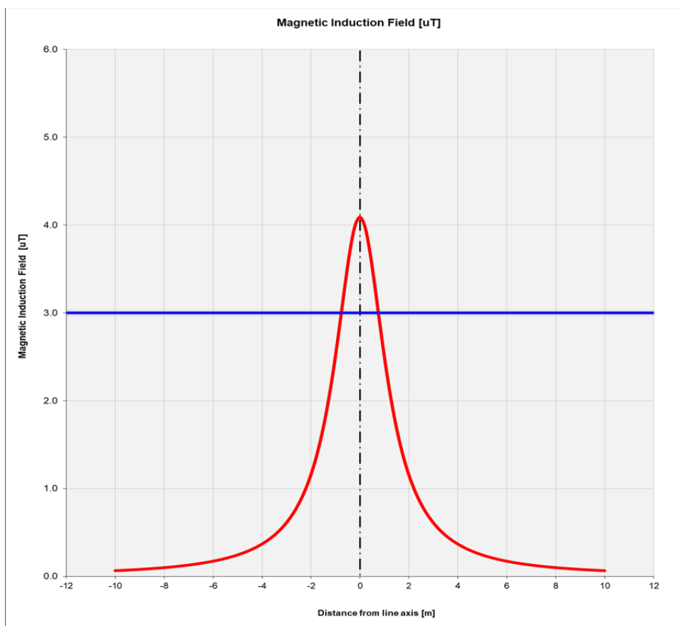
Figura 8: Andamento dell'induzione magnetica prodotta dalla linea in cavo AT calcolata a livello del suolo
