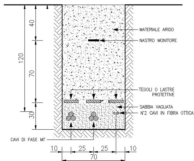
Figura 1: Tipici di posa cavi MT con n°1 linee su terreno vegetale
