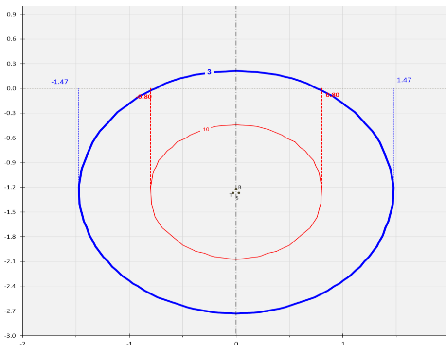
Figura 7: Andamento dell'induzione magnetica prodotta dalla linea in cavo AT calcolata a livello del suolo
