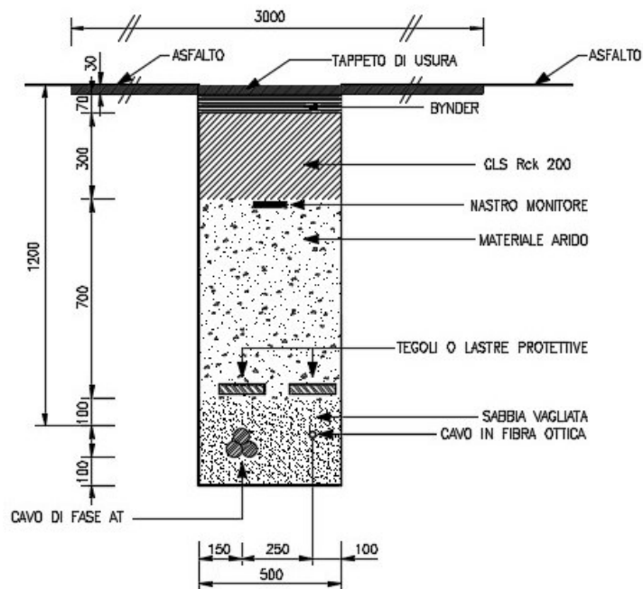
Figura 3: Tipici di posa cavo AT con n°1 linea su viabilità asfaltata
