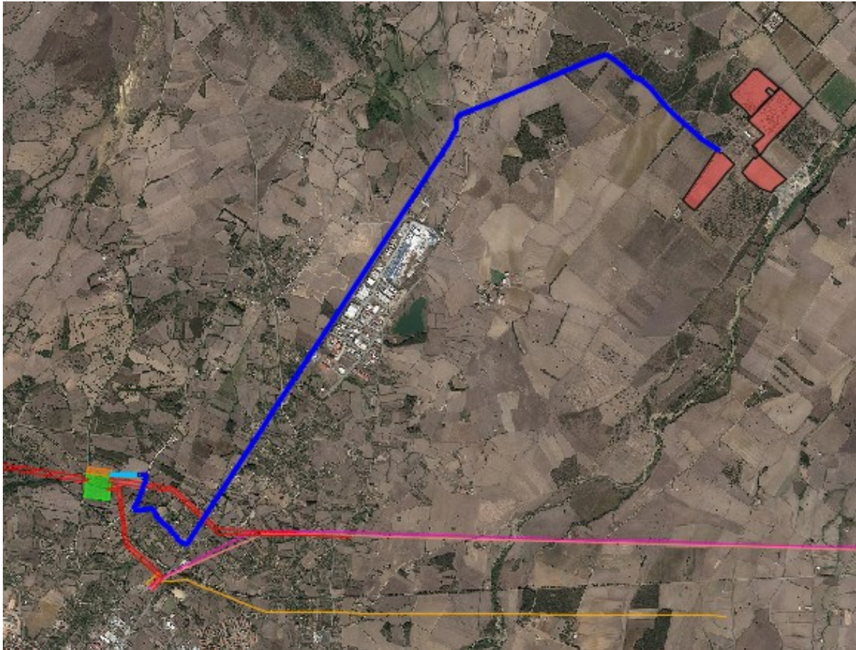
Figura 1: Tracciato degli elettrodotti MT
