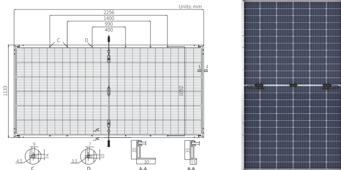
Figura 4.1 - Modulo fotovoltaico tipo: LR5-72HBD-545M
