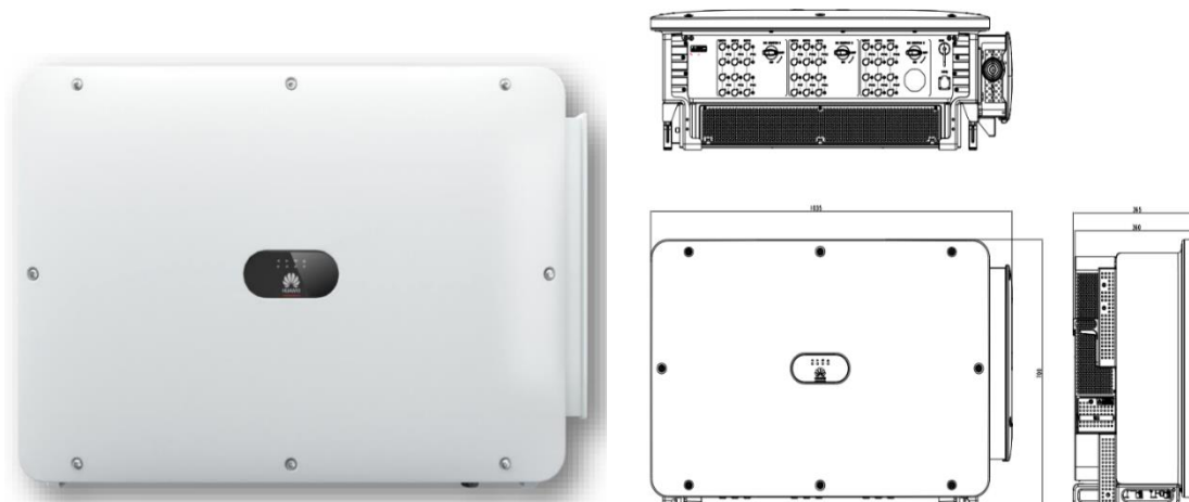
Figura 4.4 – Modulo inverter di stringa tipo SUN2000-215KTL-H0.
