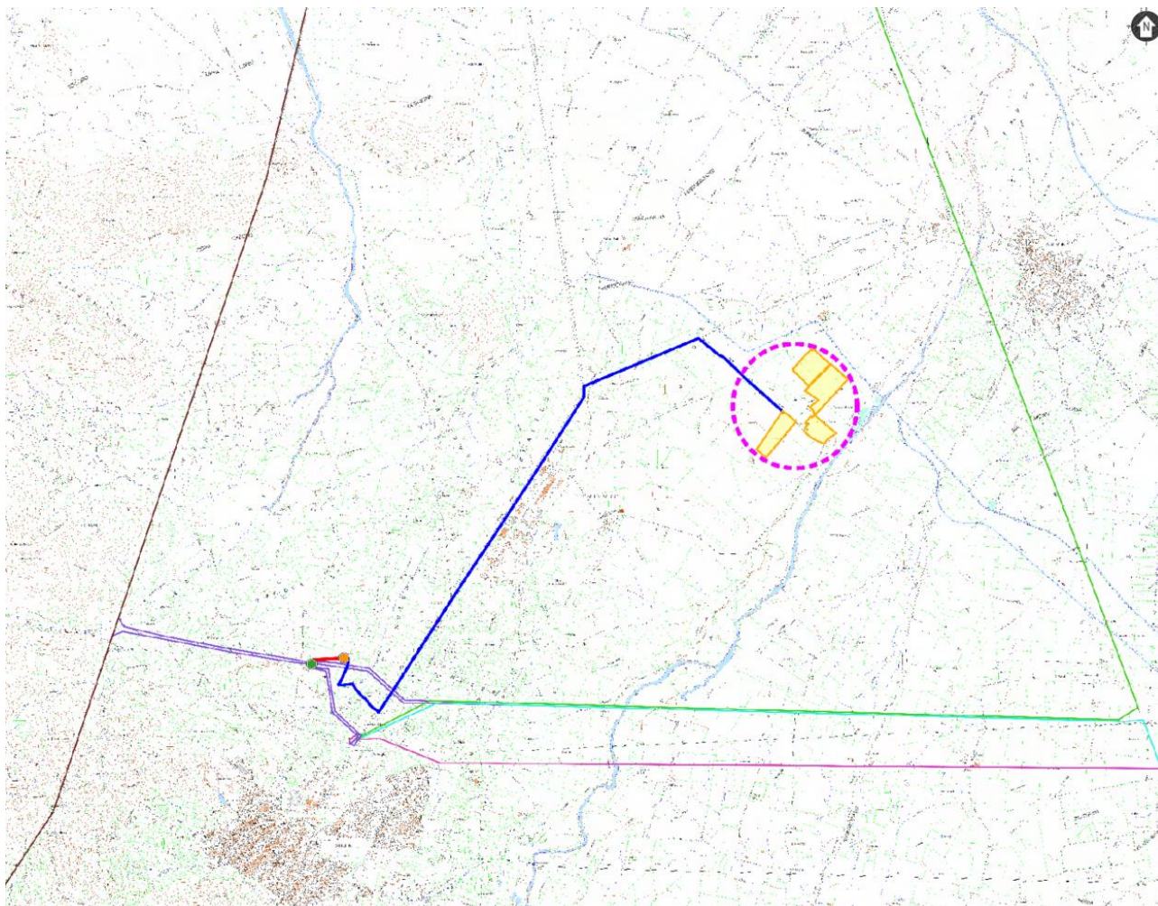
Figura 3.1: Collegamento MT alla Stazione di utenza
