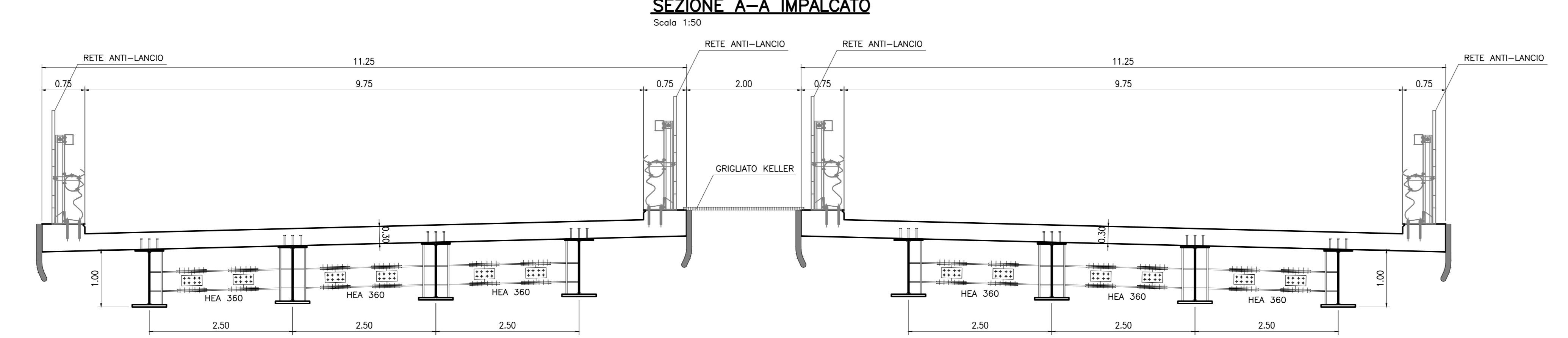
SEZIONE A-A IMPALCATO Scala: 1:50
