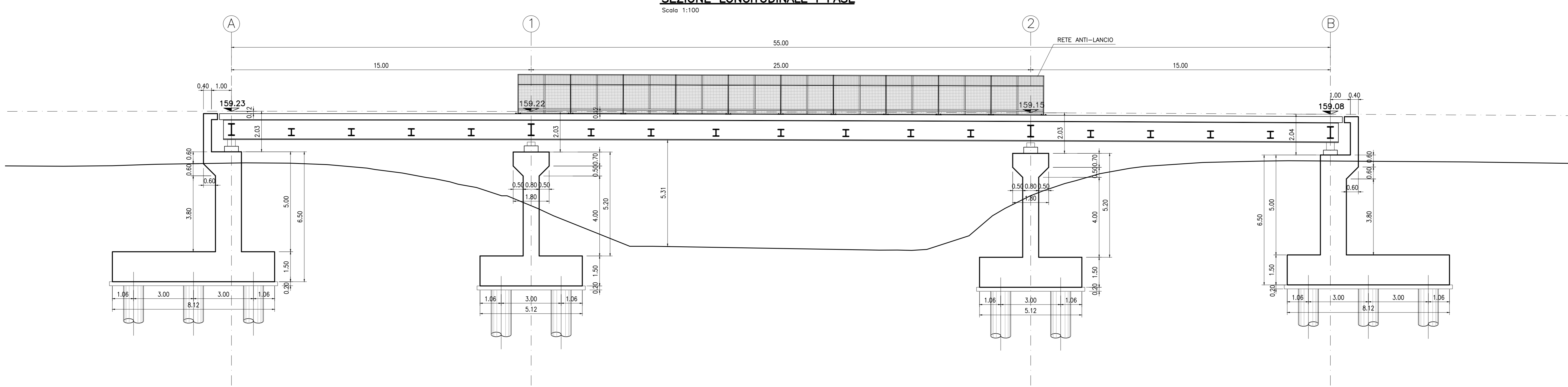
SEZIONE LONGITUDINALE I FASE Scala: 1:100
