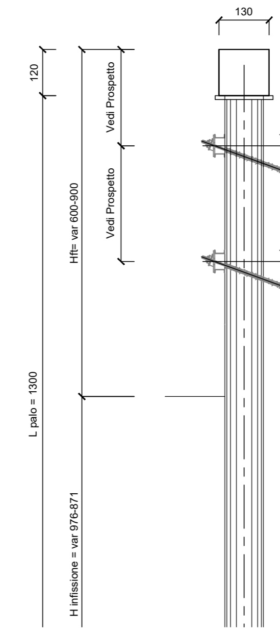
PARTICOLARE TIRANTE A TREFOLI scala 1:10
