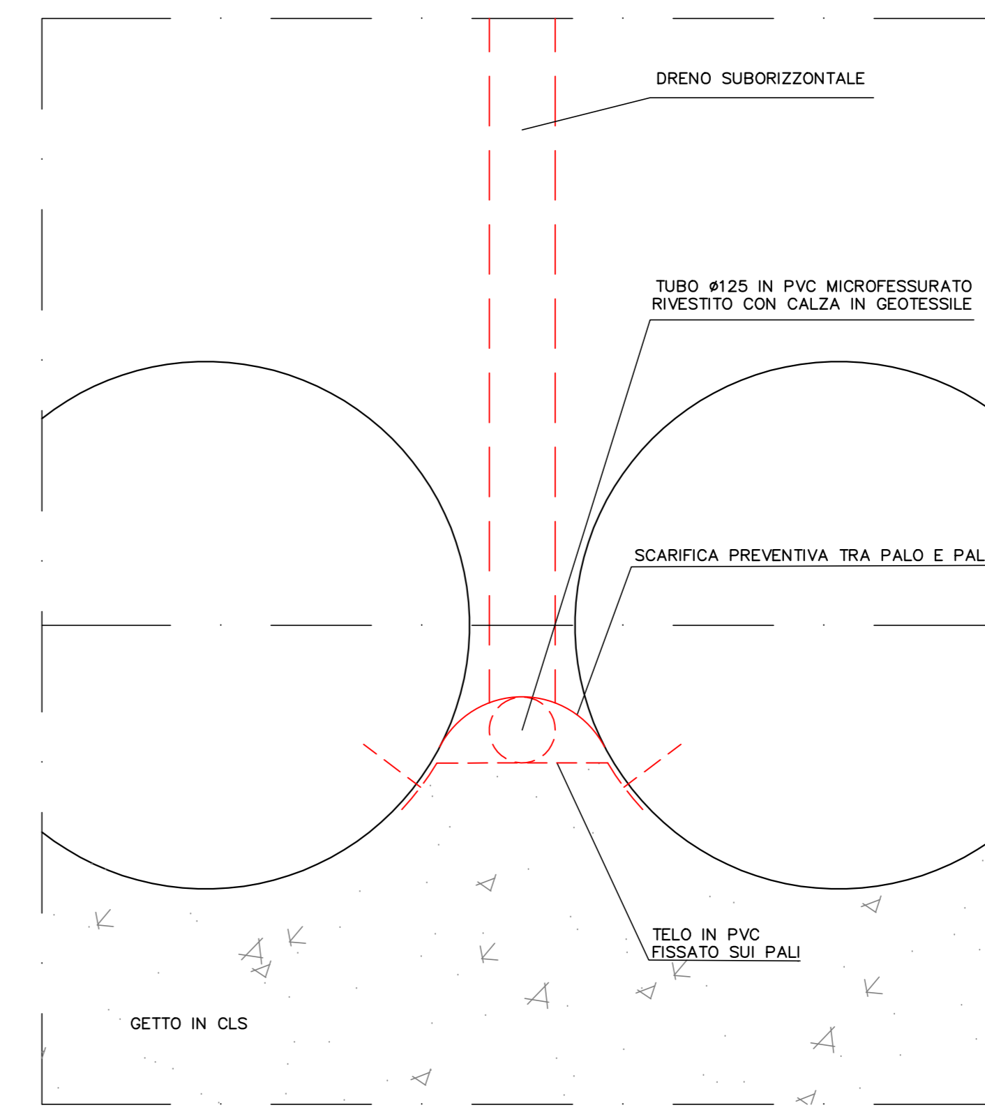
DETTAGLIO scala 1:10
