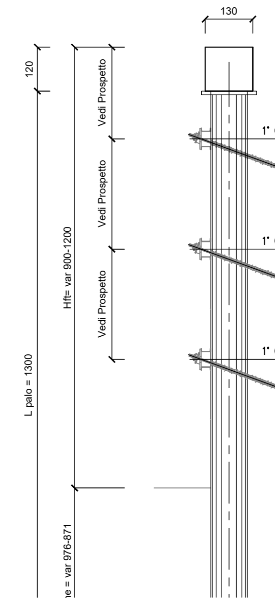
SEZIONE TIPO D
