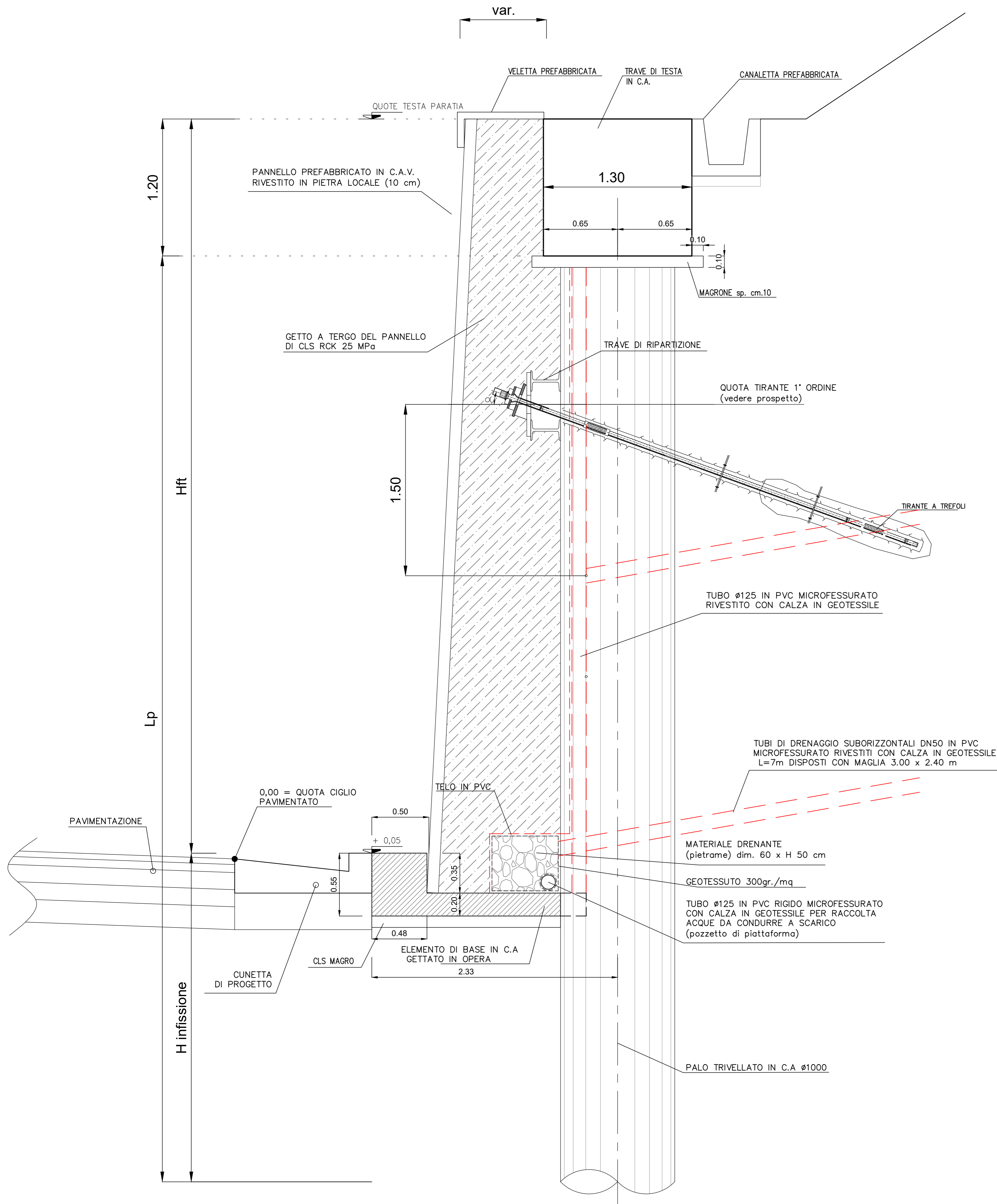
SEZIONE TIPO PARATIA DI PALI Ø1000 scala 1:20
