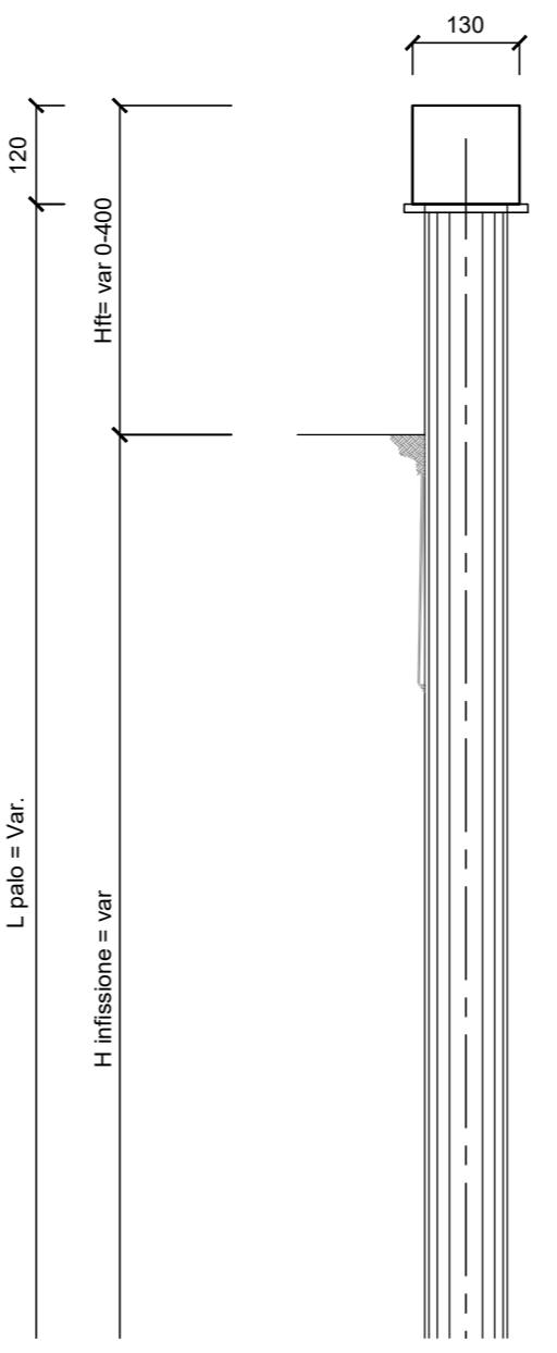
SEZIONE TIPO A
