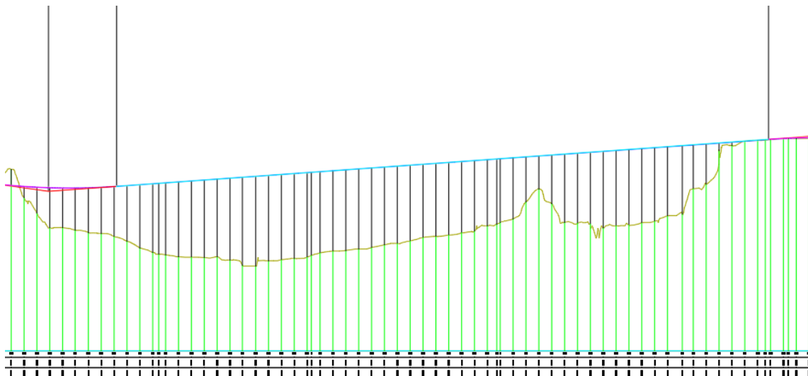
Fig. 10 -. Profilo viadotto Volturno
