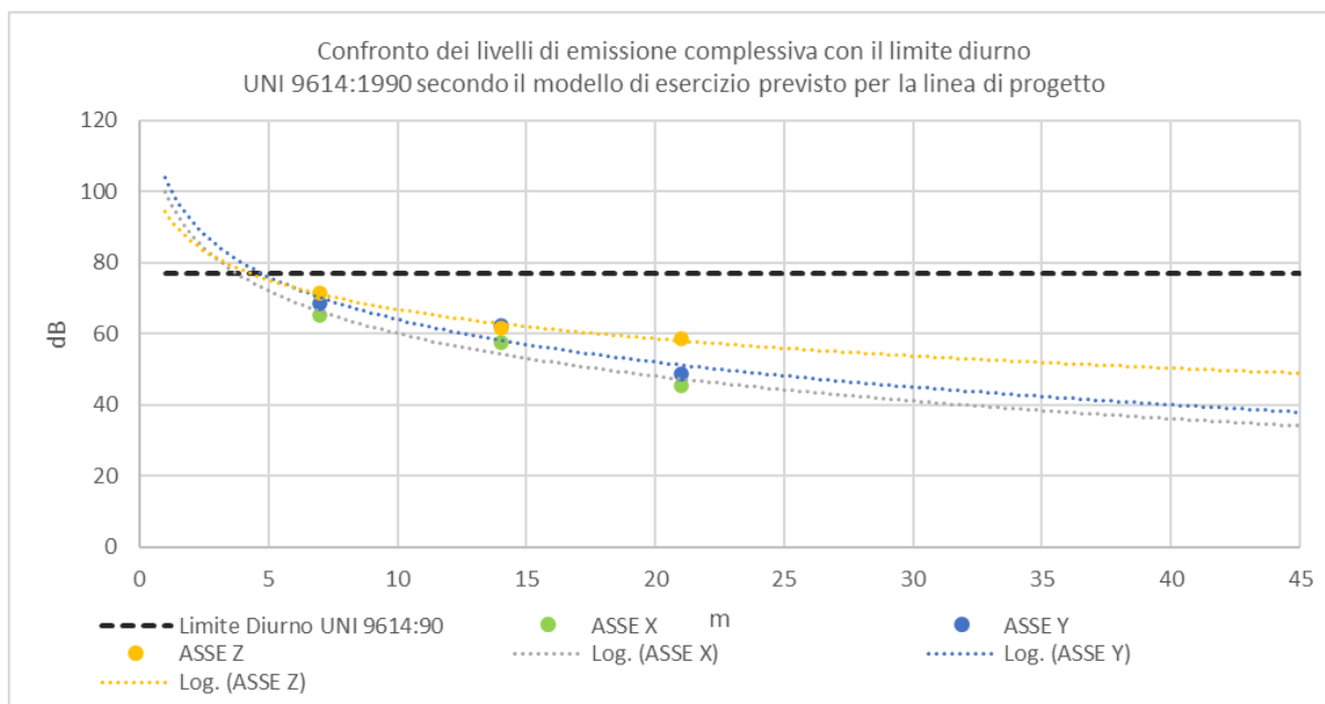
Figura 6-1 Confronto dei livelli di emissione complessiva all'interno degli edifici con i limiti UNI 9614:1990 in funzione della distanza dal binario secondo il modello di esercizio previsto – Periodo diurno.
