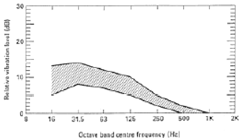
Figura 5-9 Amplificazione prodotta dai solai
