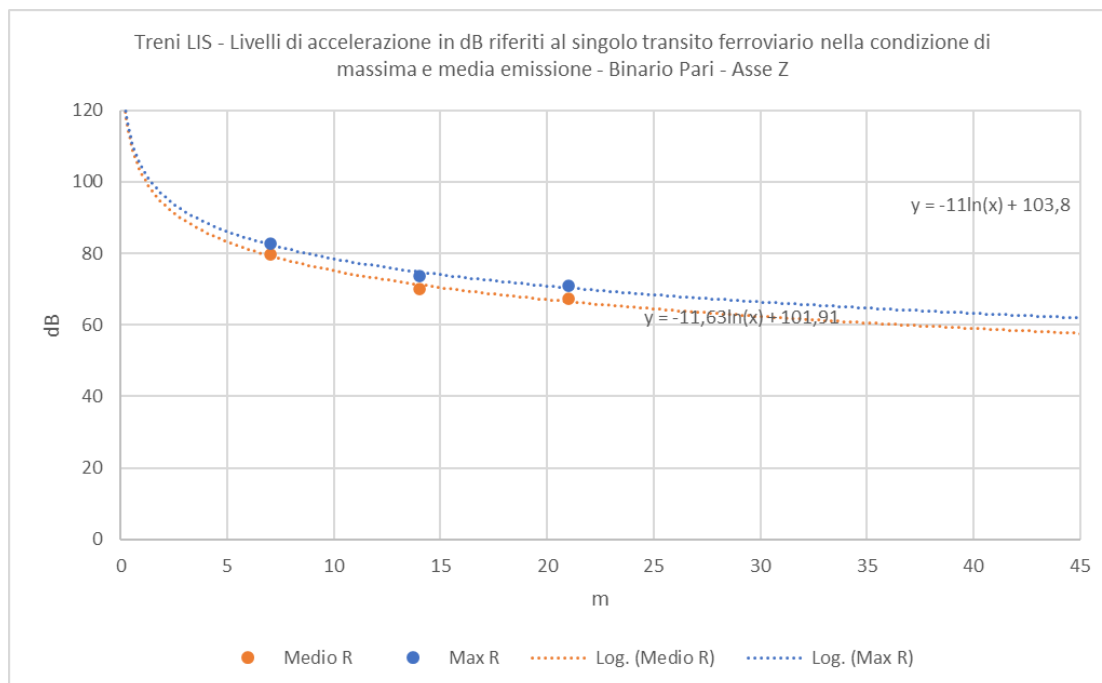
Figura 5-6 Individuazione della legge di propagazione delle vibrazioni nel terreno sulla base dei dati sperimentali lungo l'asse Z per la tipologia di treno LIS nella condizione di massima e media emissione.
