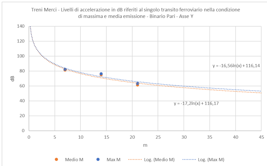
Figura 5-2 Individuazione della legge di propagazione delle vibrazioni nel terreno sulla base dei dati sperimentali lungo l'asse Y per la tipologia di treno merci nella condizione di massima e media emissione.
