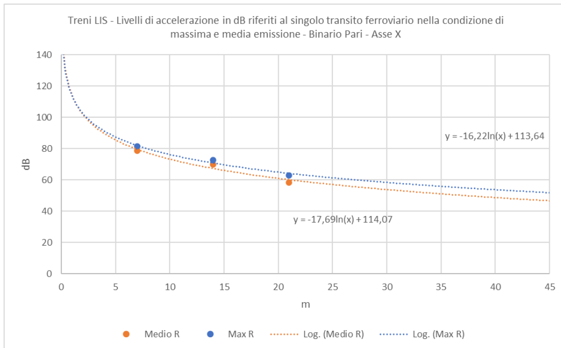
Figura 5-4 Individuazione della legge di propagazione delle vibrazioni nel terreno sulla base dei dati sperimentali lungo l'asse X per la tipologia di treno LIS nella condizione di massima e media emissione.
