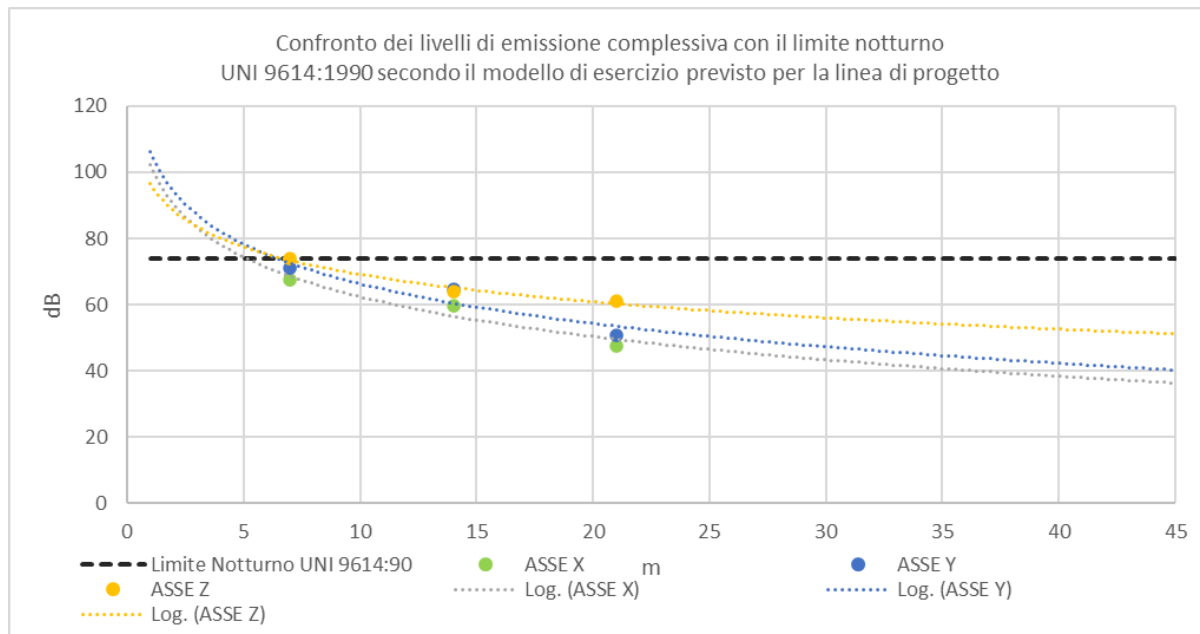
Figura 6-2 Confronto dei livelli di emissione complessiva all'interno degli edifici con i limiti UNI 9614:1990 in funzione della distanza dal binario secondo il modello di esercizio previsto – Periodo notturno.
