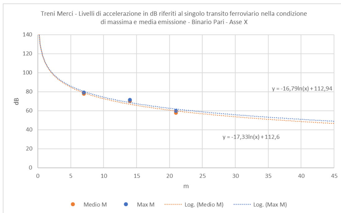
Figura 5-1 Individuazione della legge di propagazione delle vibrazioni nel terreno sulla base dei dati sperimentali lungo l'asse X per la tipologia di treno merci nella condizione di massima e media emissione.
