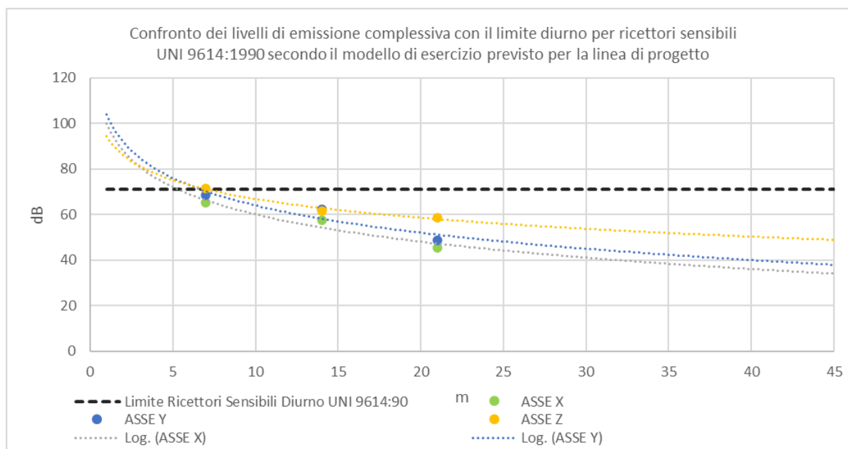
Figura 6-3 - Confronto dei livelli di emissione complessiva all'interno degli edifici sensibili con i limiti UNI 9614:1990 in funzione della distanza dal binario secondo il modello di esercizio previsto – Periodo diurno.
