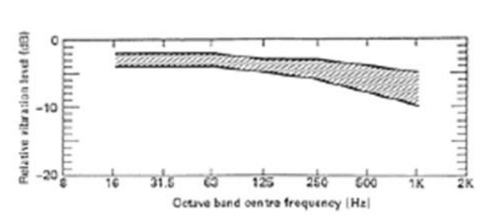
Figura 5-8 Attenuazione delle vibrazioni nel passaggio da un piano al successivo
