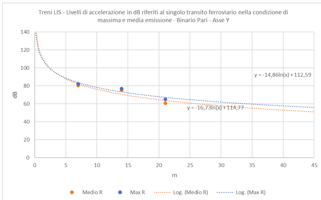
Figura 5-5 Individuazione della legge di propagazione delle vibrazioni nel terreno sulla base dei dati sperimentali lungo l'asse Y per la tipologia di treno LIS nella condizione di massima e media emissione.
