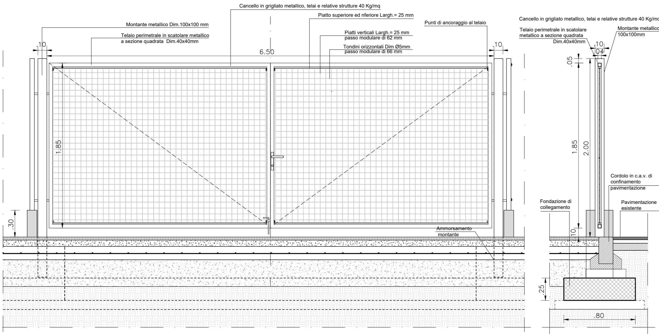
DETTAGLIO "D" Cannello metallico di accesso al piazzale 40 Kg/mq
