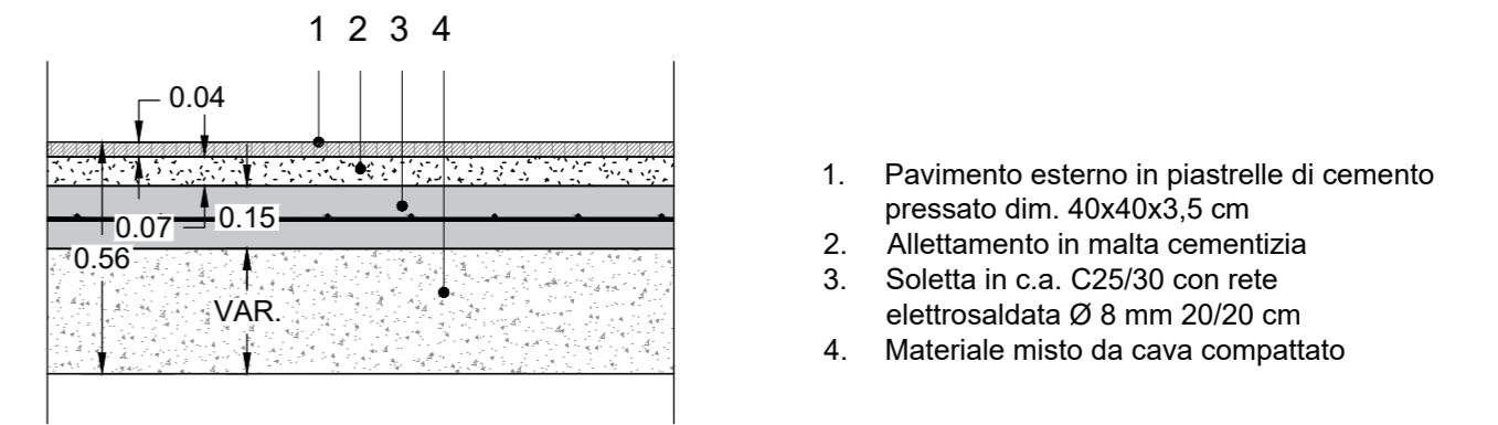
DETTAGLIO "C" - Marciapiede
