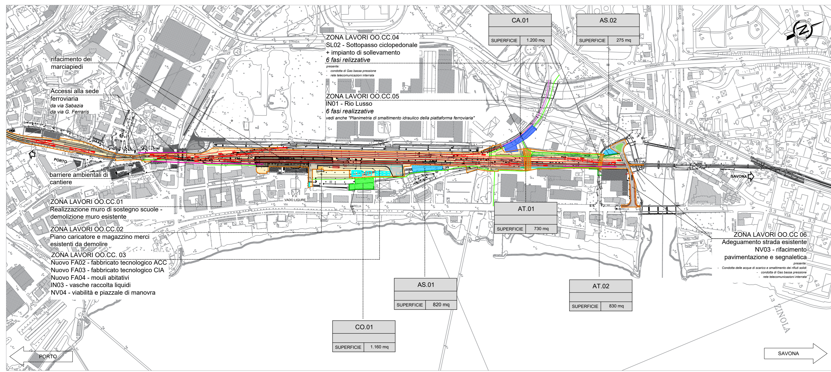
Inquadramento generale delle aree di intervento Scala 1:4000
