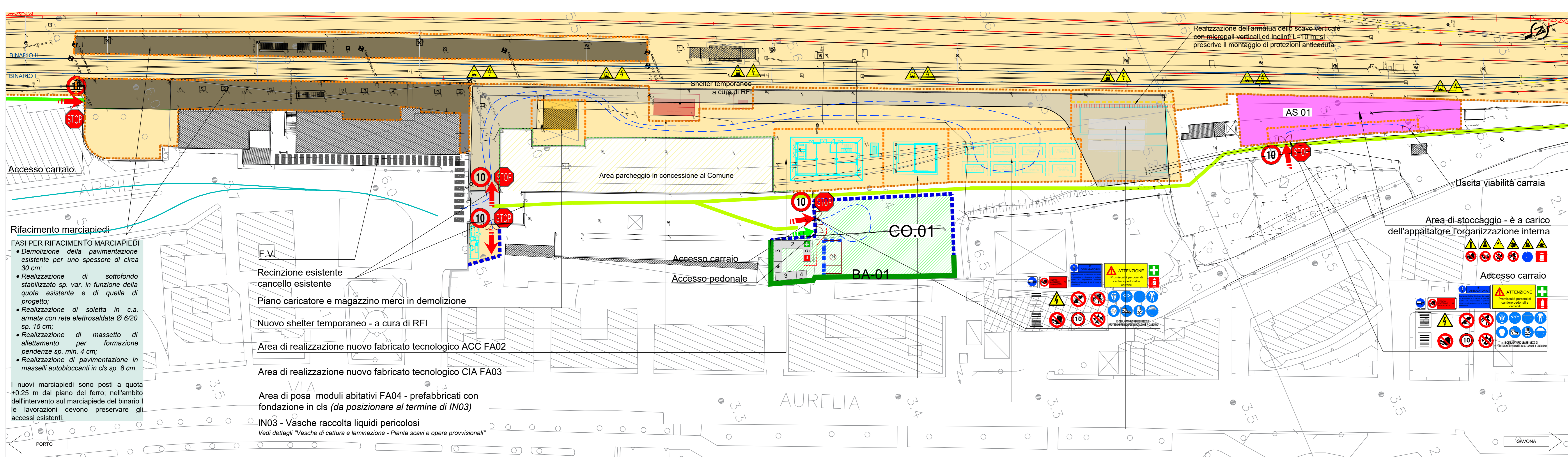
Dettaglio aree di lavoro e cantieri CO.01 e AS.01 Scala 1:500
