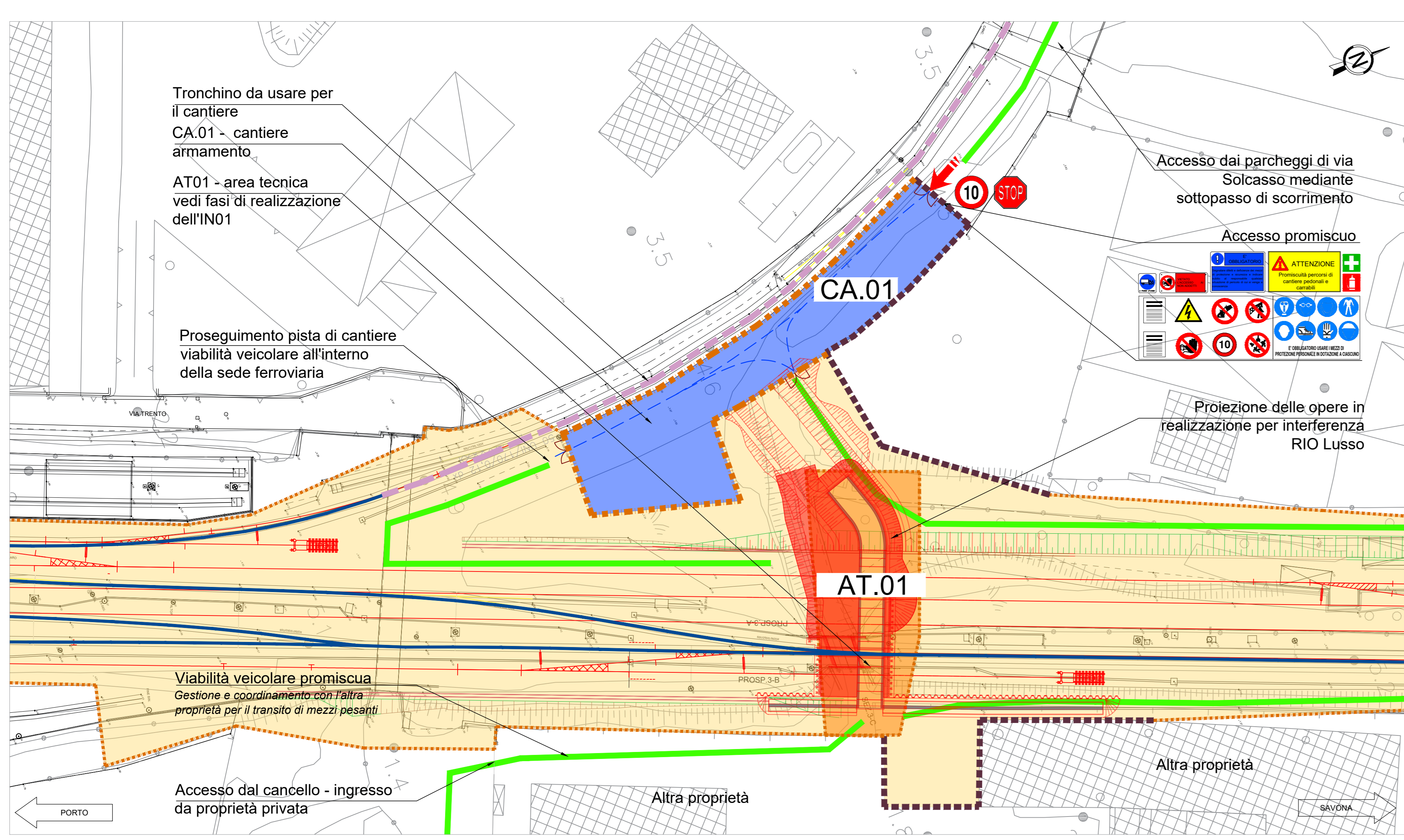
Dettaglio cantieri CA.01 e AT.01 Scala 1:500
