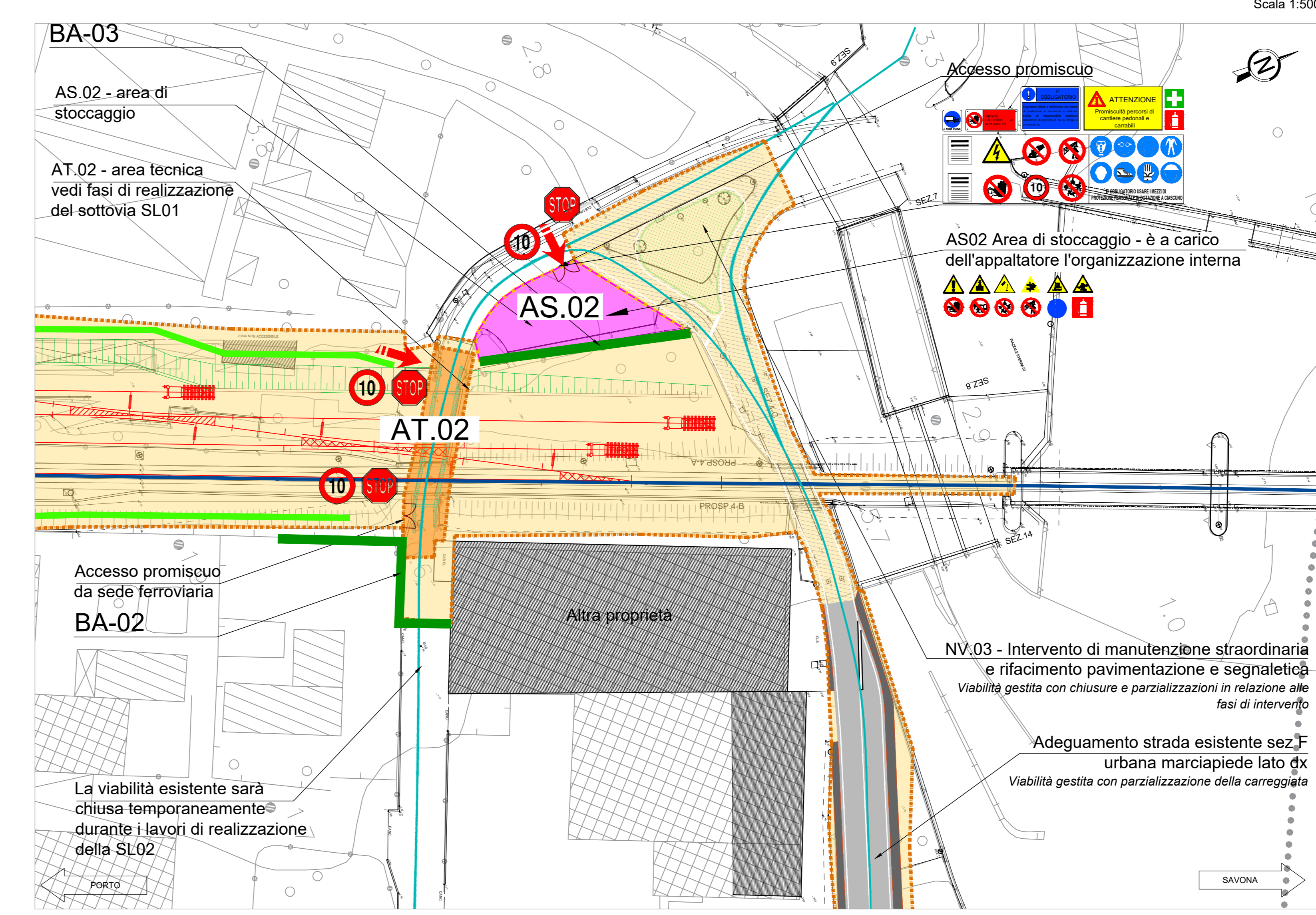
Dettaglio cantieri AS.02 e AT.02 Scala 1:500
