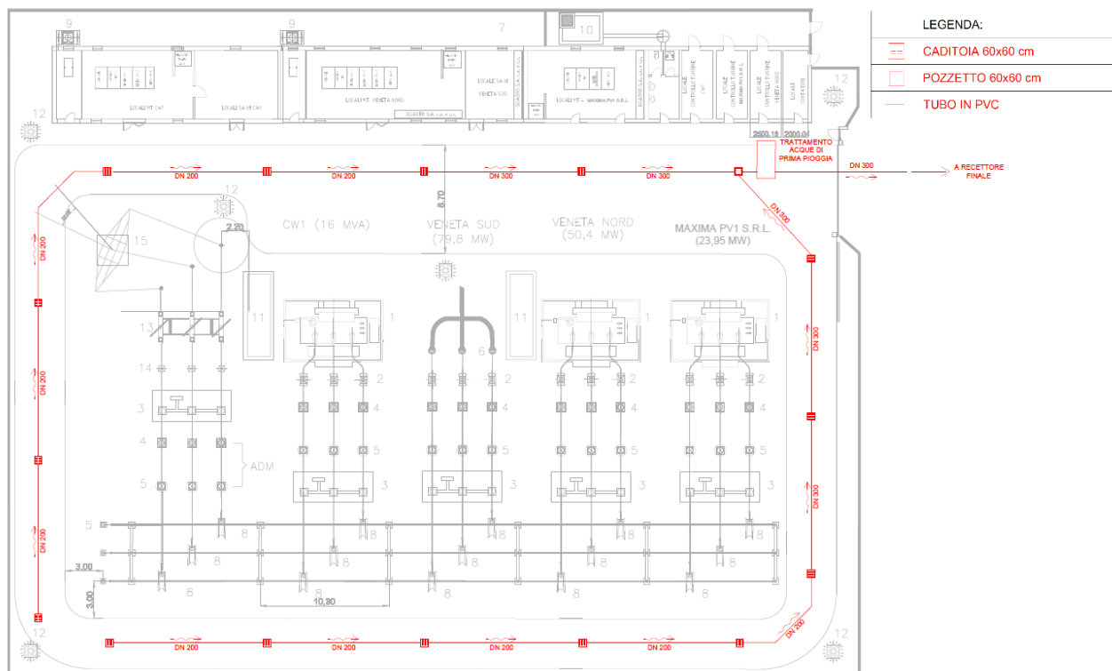
Regimentazione acque meteoriche SSEU
