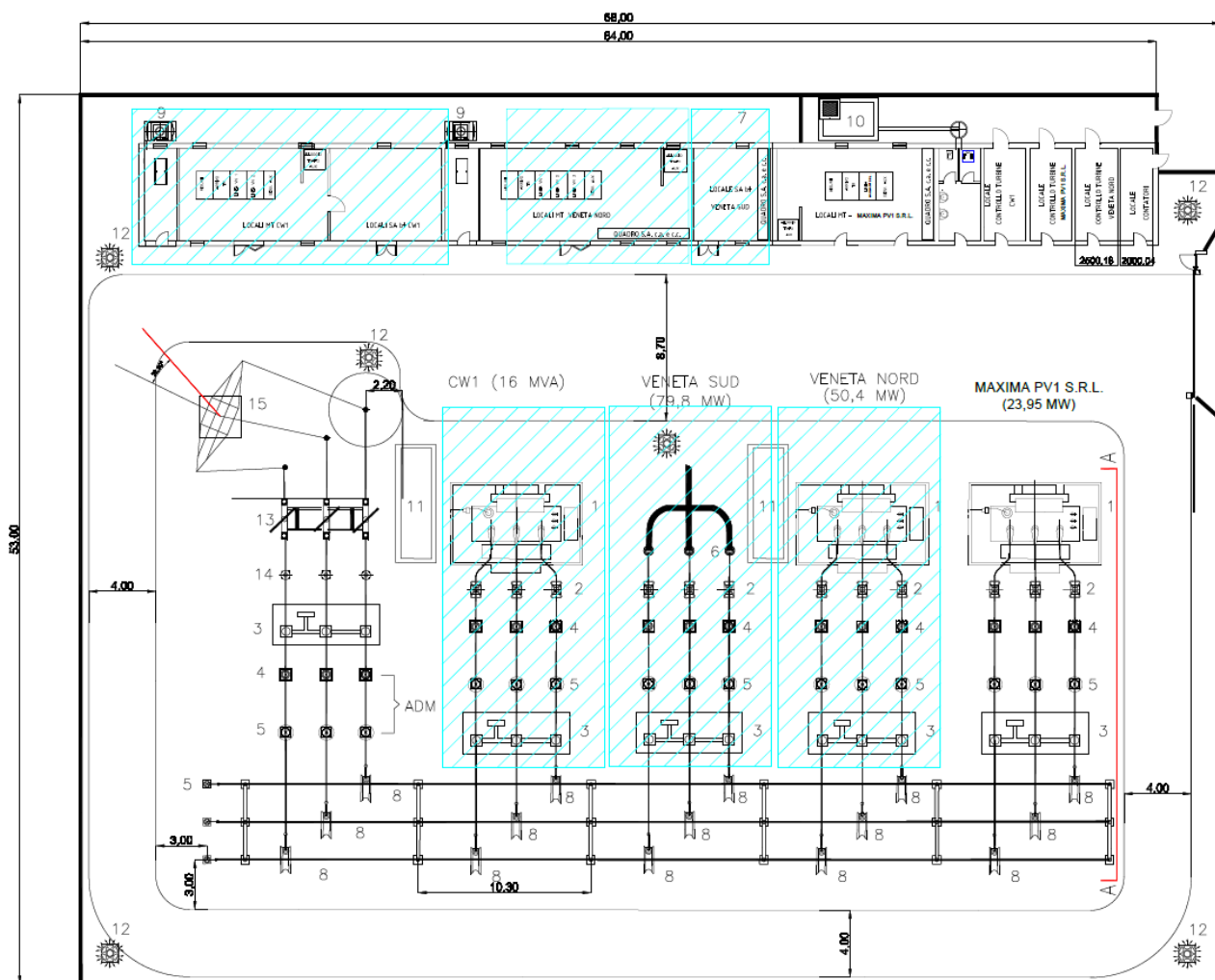
Planimetria elettromeccanica SSEU
