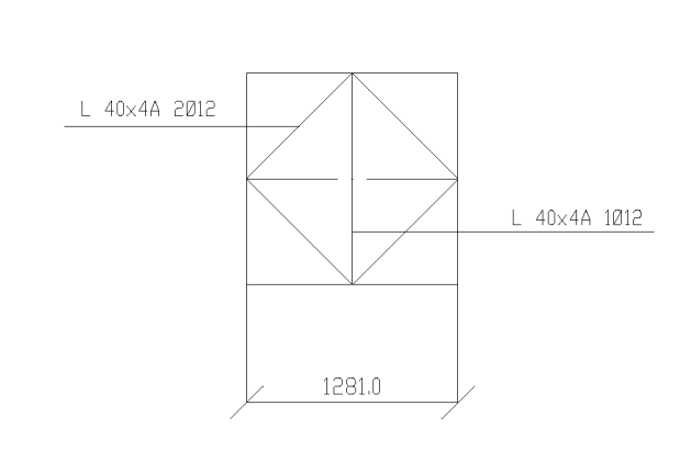
SEZIONE A-A
