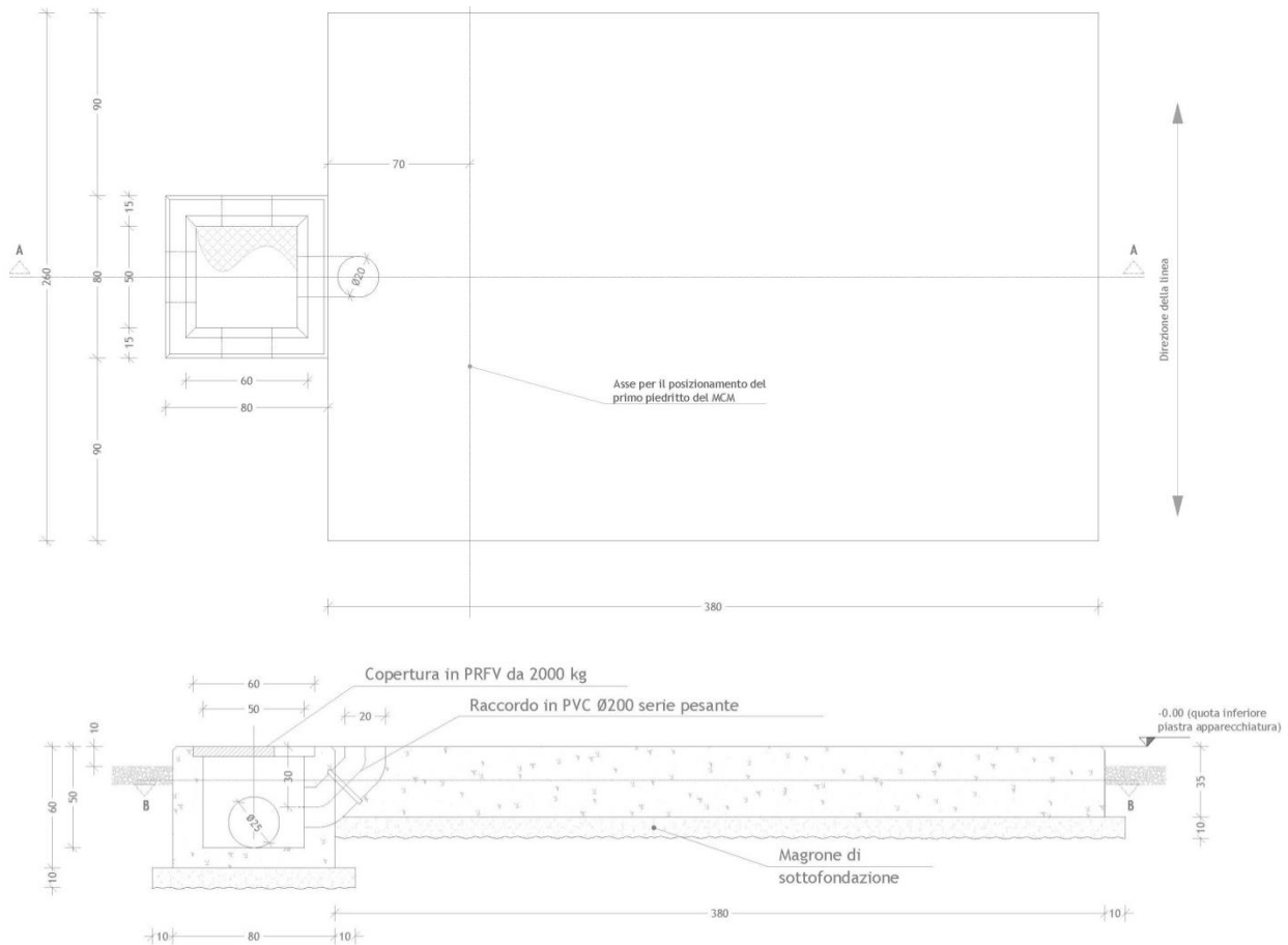
Fig. Pianta e sezione fondazione per MCM
