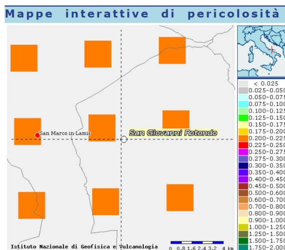
Mappa di pericolosità sismica e relativa legenda per i comuni di San Giovanni Rotondo e San Marco in Lamis
