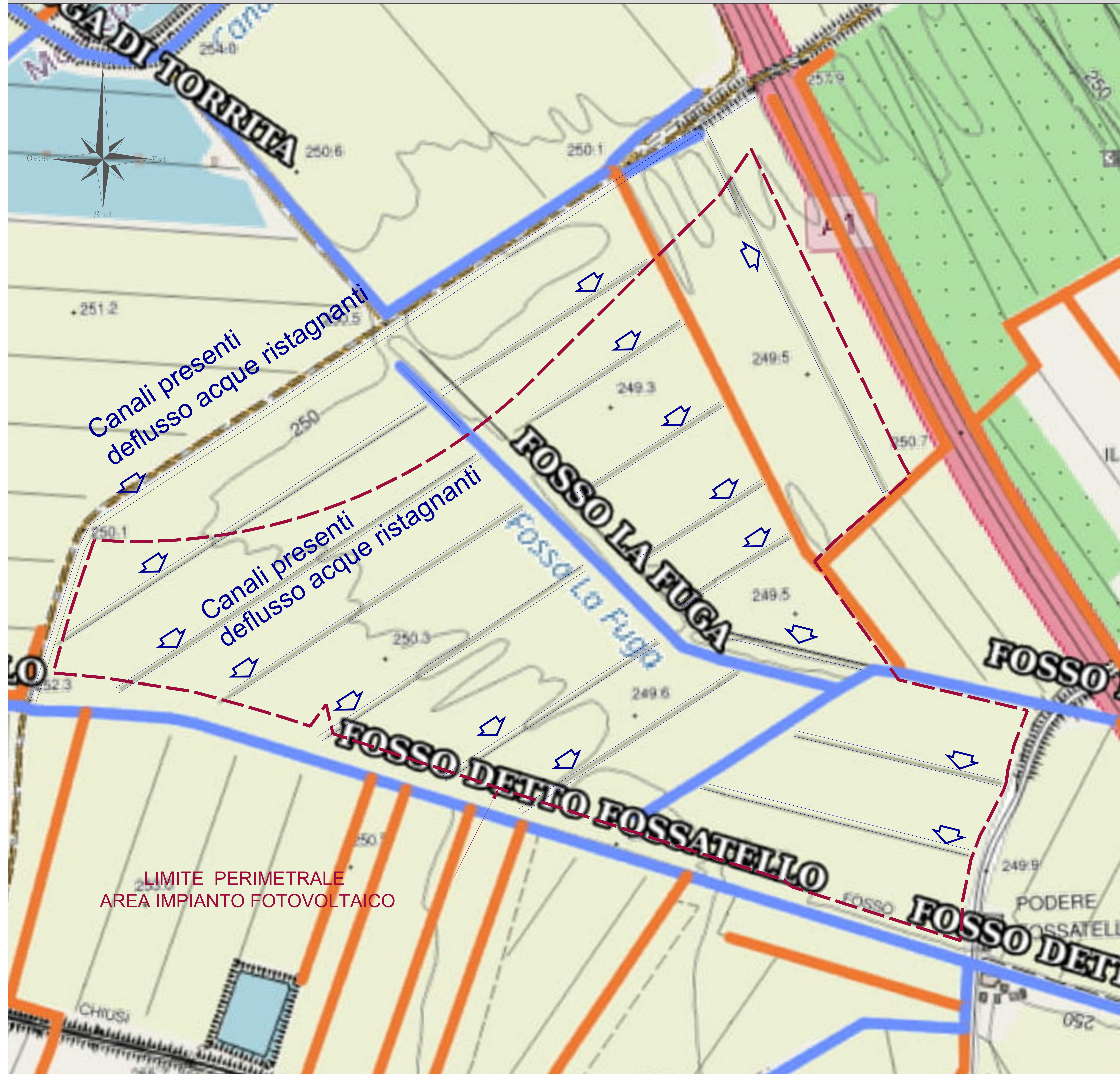
INQUADRAMENTO SU TAVOLE " RETICOLO IDROGRAFICO E DI GESTIONE "; REGIONE TOSCANA DCR 28/2020 - CANALI AREA DEDICATA IMP. FOTOVOLTAICO ; SITUAZIONE ANTE OPERAM SCALA:1:2000
