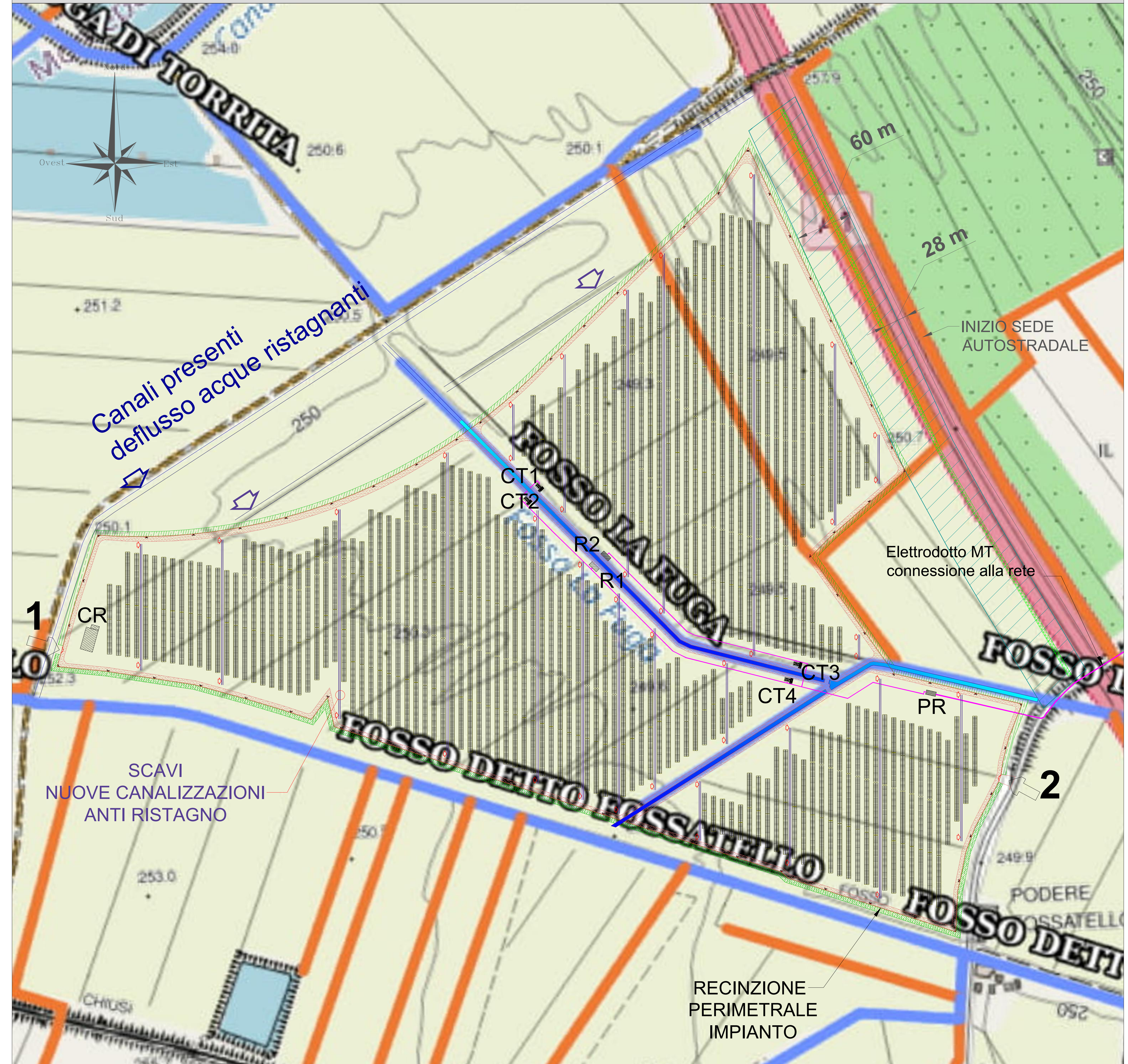
INQUADRAMENTO SU TAVOLE RETICOLO IDROGRAFICO E DI GESTIONE ; REGIONE TOSCANA DCR 28/2020 - POST OPERAM IMPIANTO FOTOVOLTAICO, NUOVE CANALIZZAZIONI ANTIRISTAGNO SCALA:1:2000
