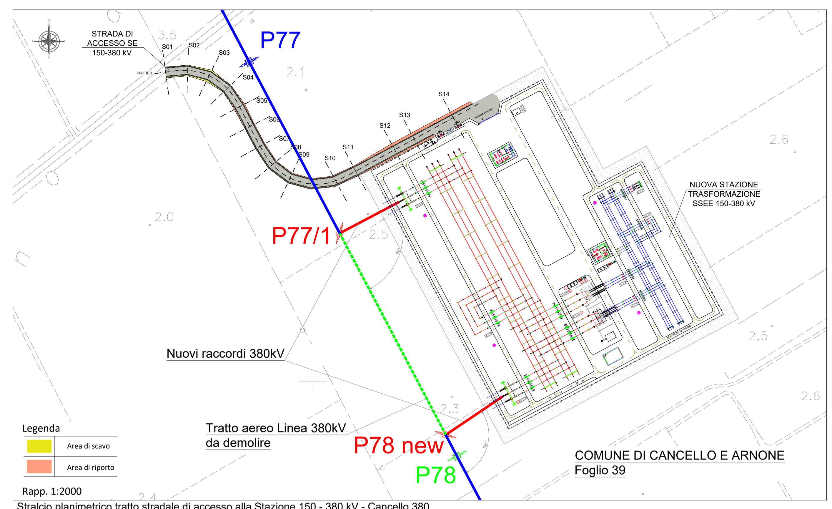
Stralcio planimetrico tratto stradale di accesso alla Stazione 150 - 380 kV - Cancellorotondo
