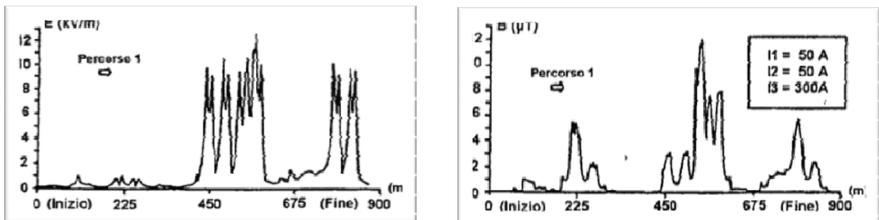
Figura 10 Risultati della misura dei campi elettrici e magnetici effettuate lungo le vie interne della sezione a 380 kV della stazione riportata in fig. 9
