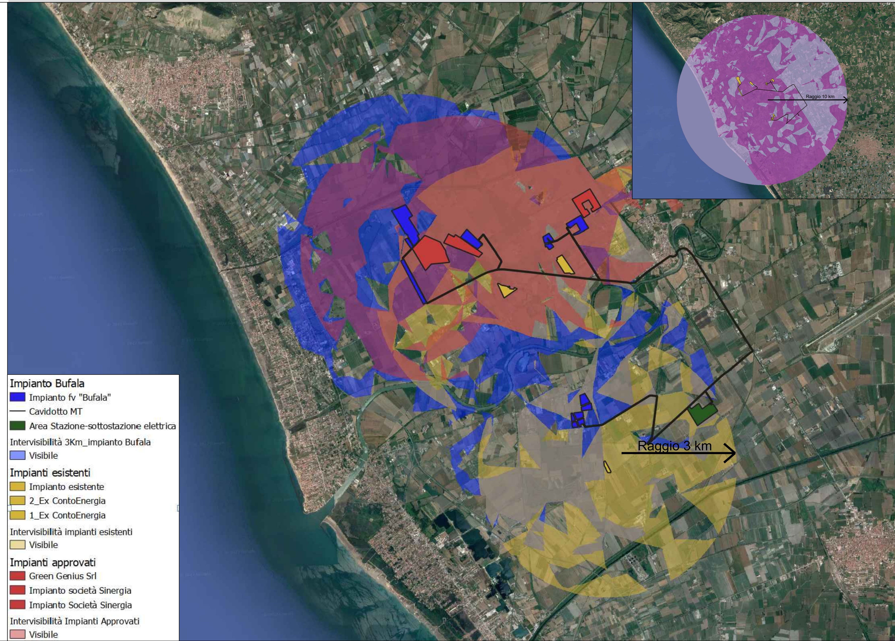
Analisi Intervisibilità impianto Bufala, impianti esistenti e impianti approvati e non ancora realizzati
