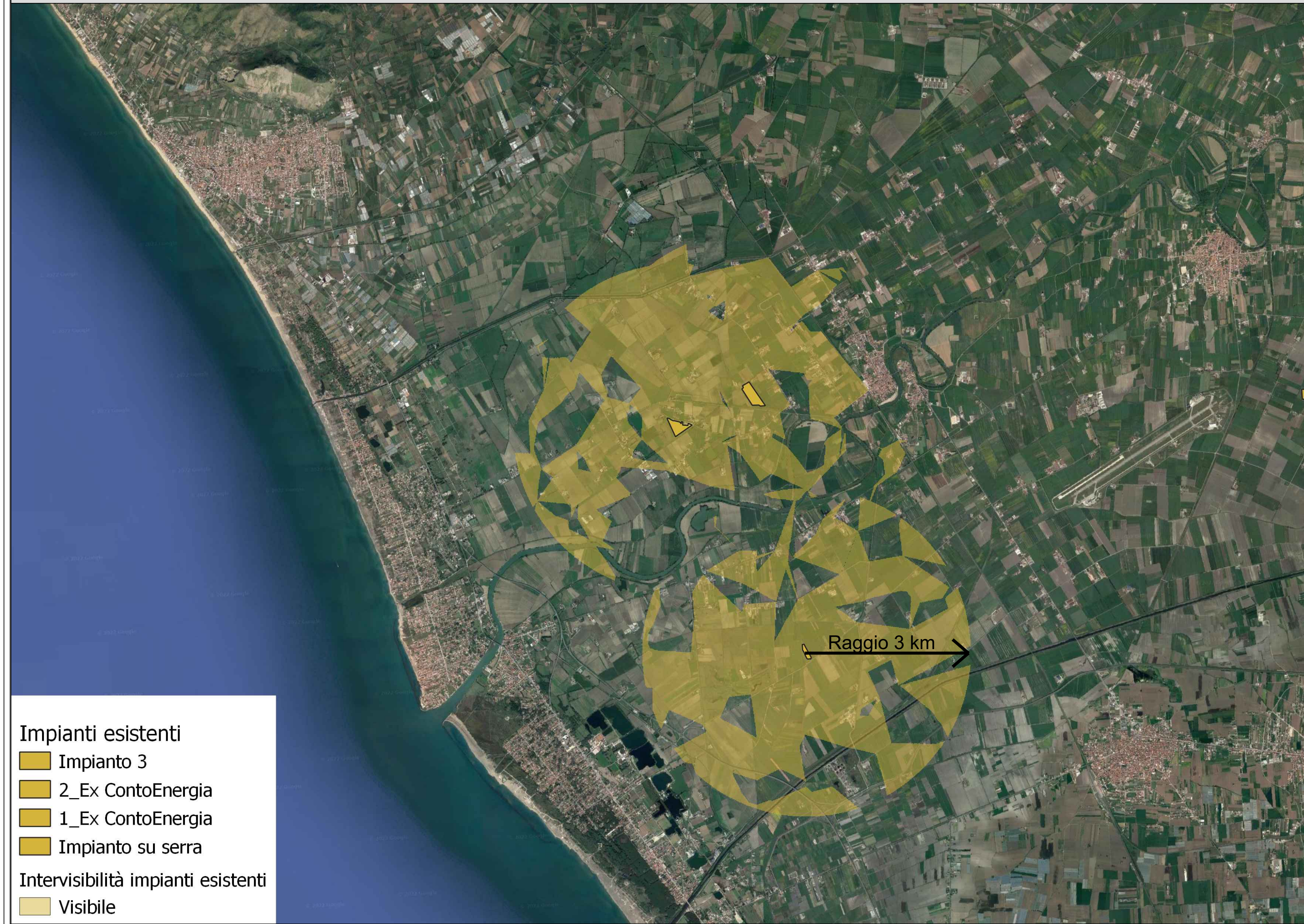
Analisi Intervisibilità impianti esistenti
