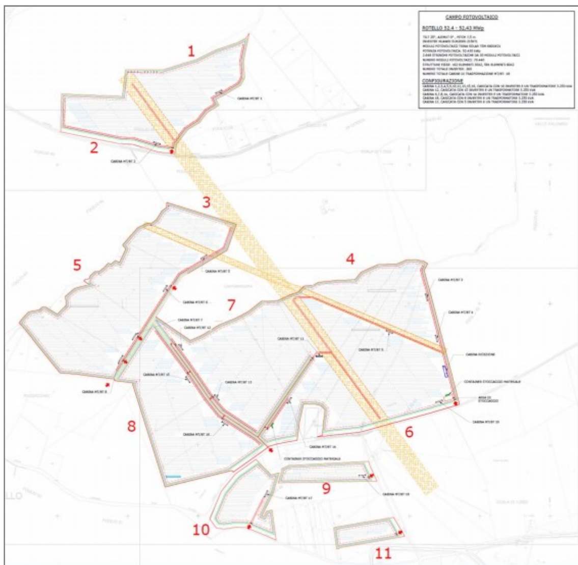
Figura 5-1: Layout impianto
