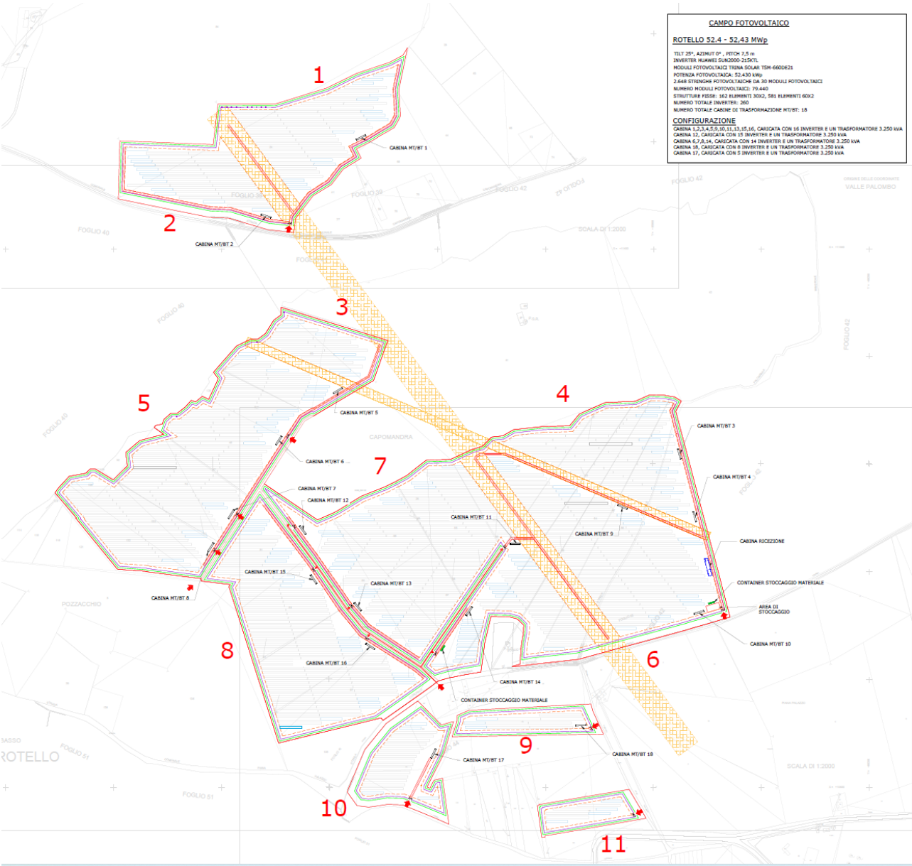
Fig. 3 - Layout di impianto
