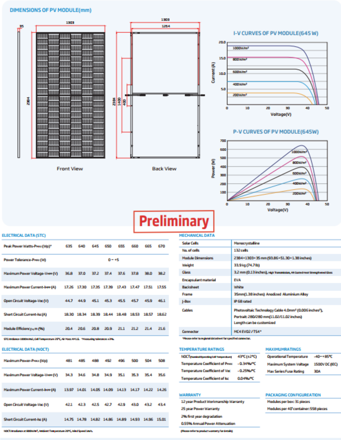
Fig. 4 - Dimensioni, specifiche tecniche e prestazionali pannelli fotovoltaici Trina Solar
