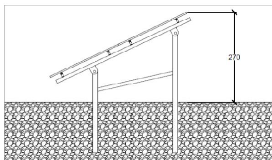
Fig. 5 - Struttura di supporto moduli
