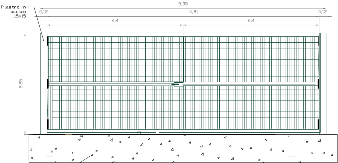
Fig. 13 – Cannello a doppia anta
