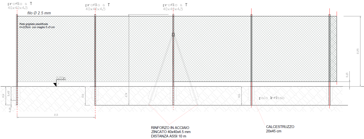
Fig. 12 – Recinzione perimetrale
