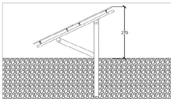
Fig. 5 - Struttura di supporto moduli
