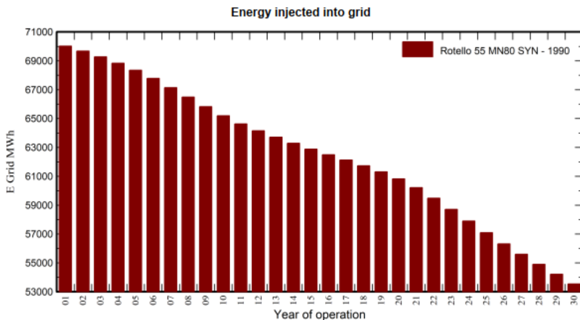
Fig. 25 – Producibilità dell’impianto con degrado moduli (30 anni)
