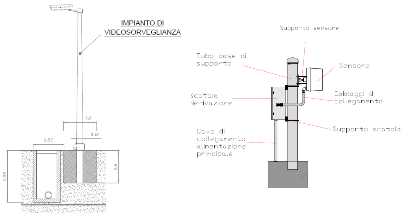
Fig. 19 – Sistema antintrusione
