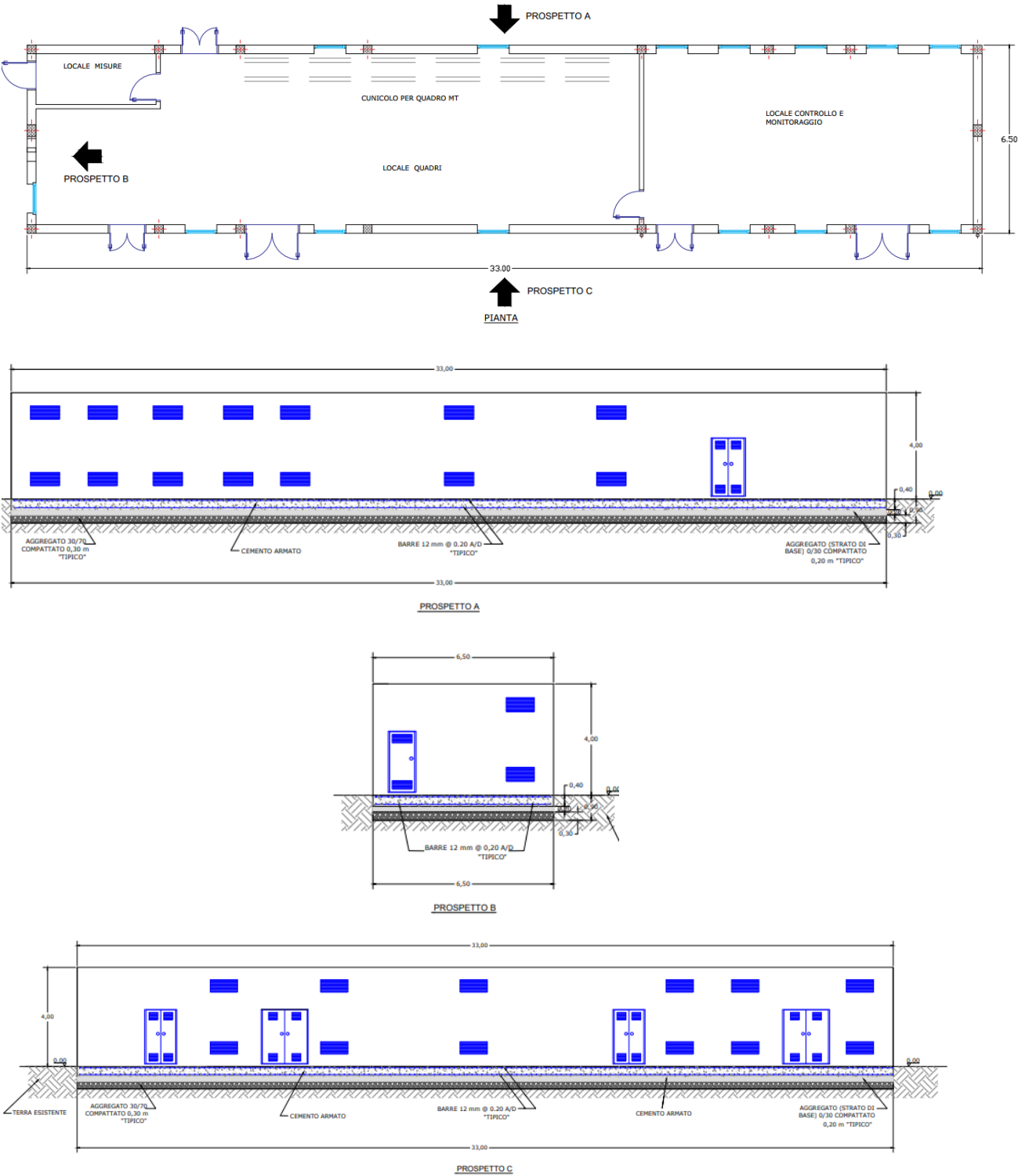
Fig. 15 - Cabina di ricezione
