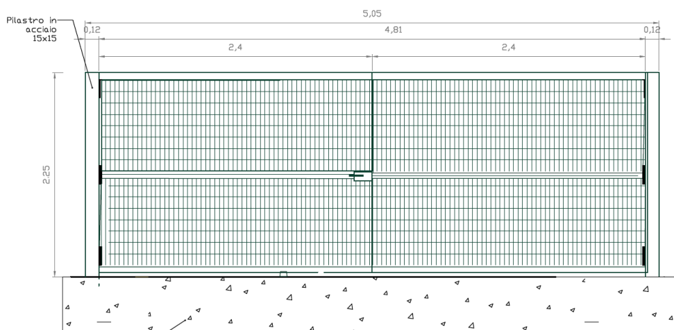
Fig. 19 – Cannello a doppia anta
