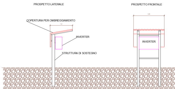
Fig. 4 - Tipico struttura supporto inverter
