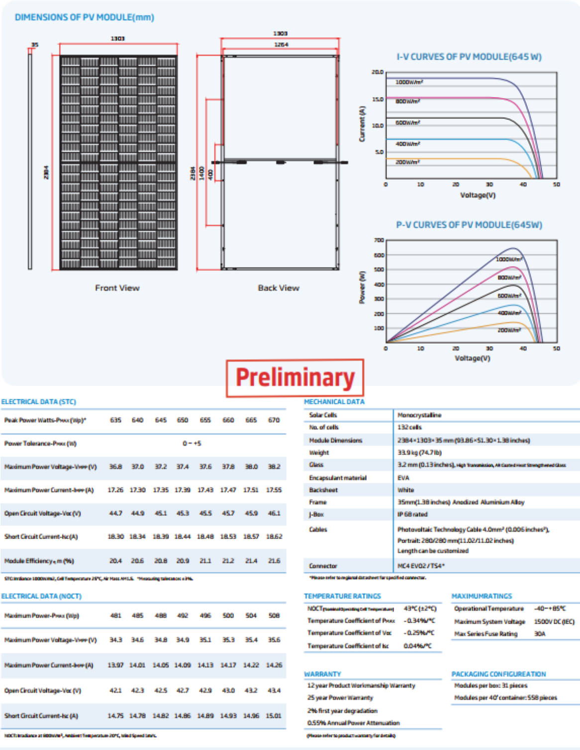
Fig. 1 - Dimensioni, specifiche tecniche e prestazionali pannelli fotovoltaici Trina Solar
