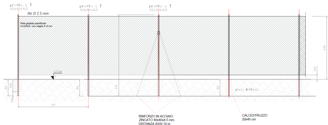
Fig. 18 – Particolare della recinzione
