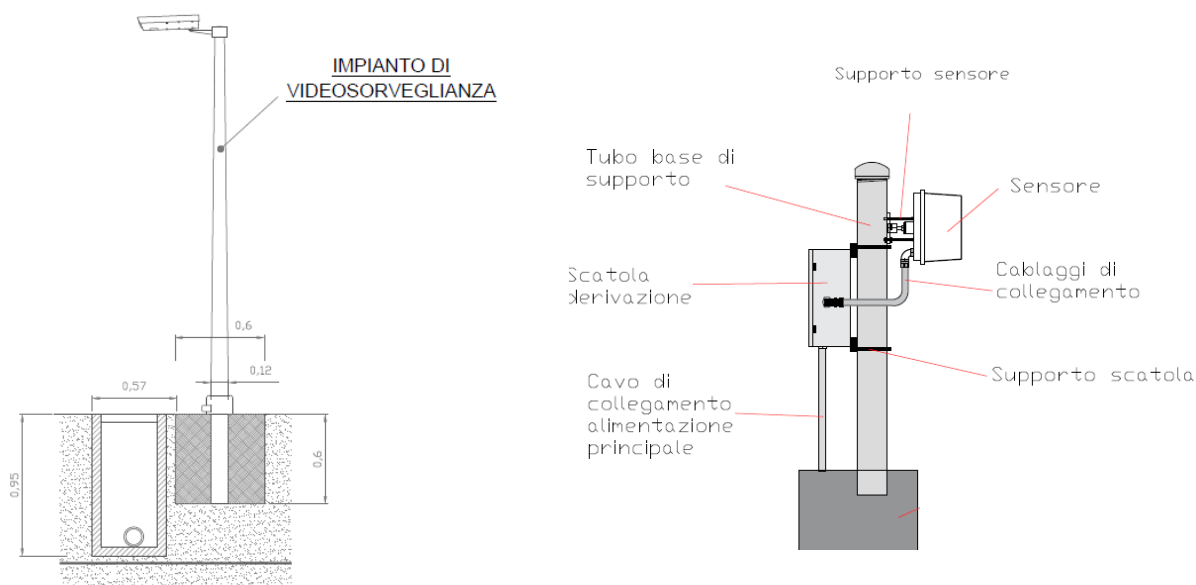
Fig. 21 – Sistema antintrusione
