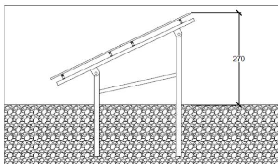
Fig. 2 - Struttura di supporto moduli
