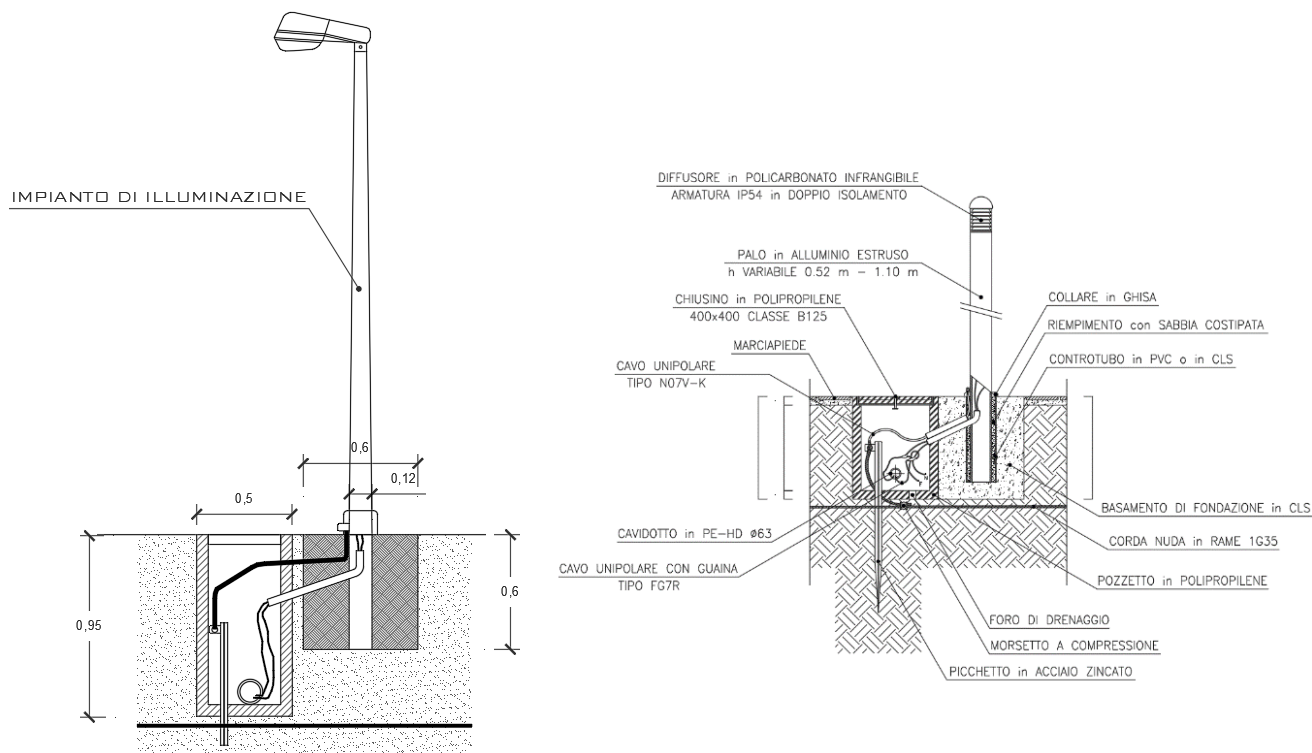
Fig. 22 – Sistema di illuminazione
