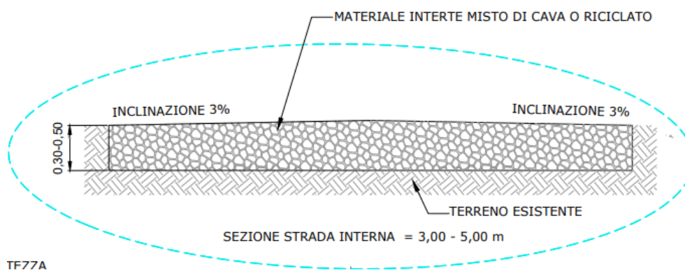
Fig. 20 – Sezione strada perimetrale
