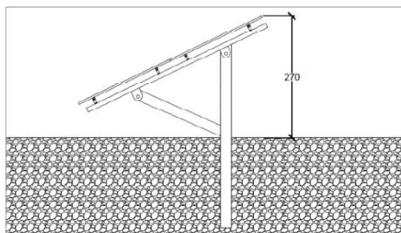
Fig. 2 - Struttura di supporto moduli
