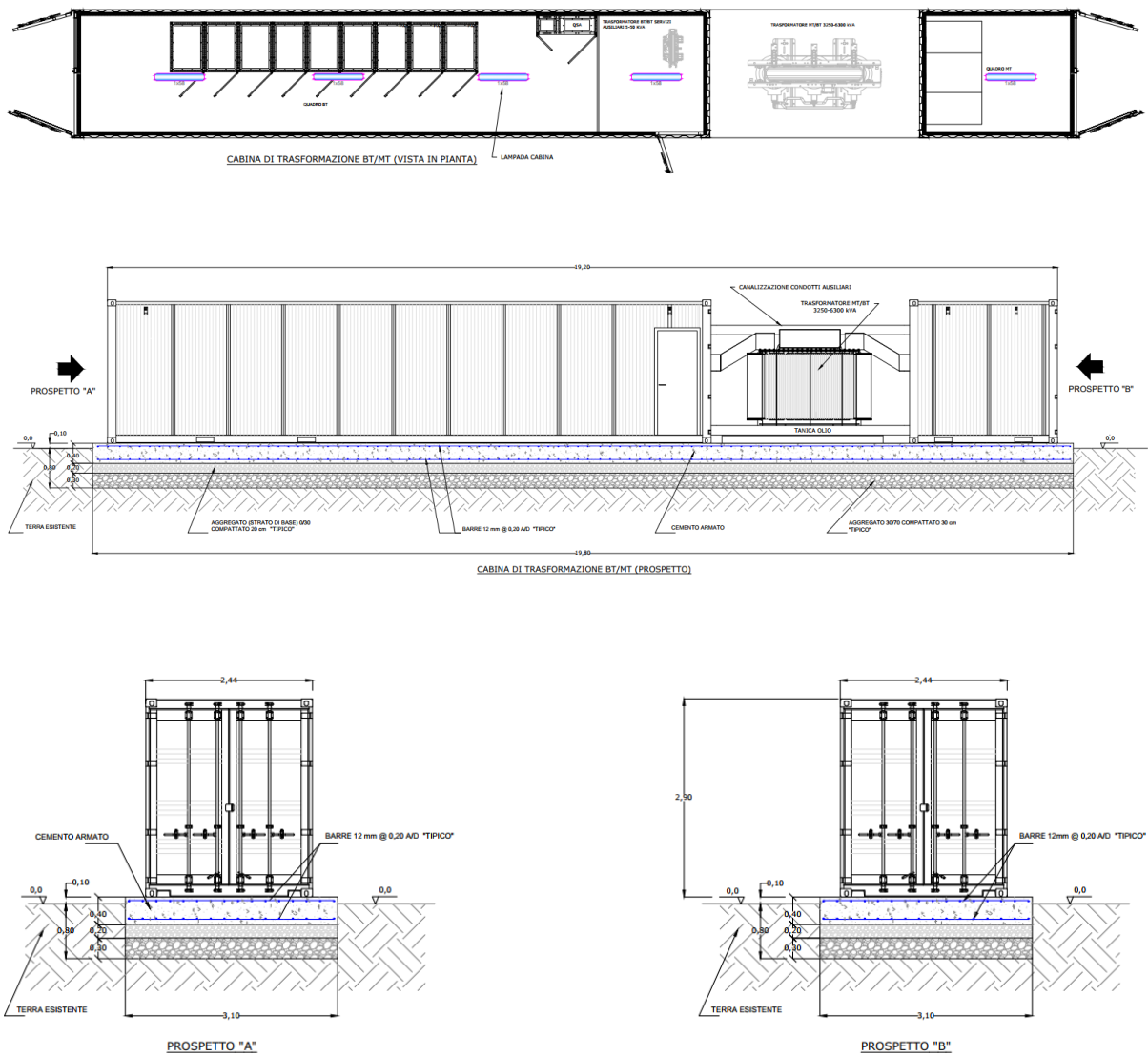
Fig.14 – Cabina di trasformazione BT/MT
