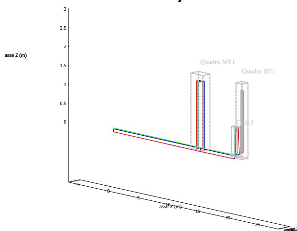
Fig.6 - Modello spaziale cablaggi nelle cabine di trasformazione MT/BT
