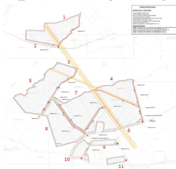
LAY-OUT IMPIANTO
