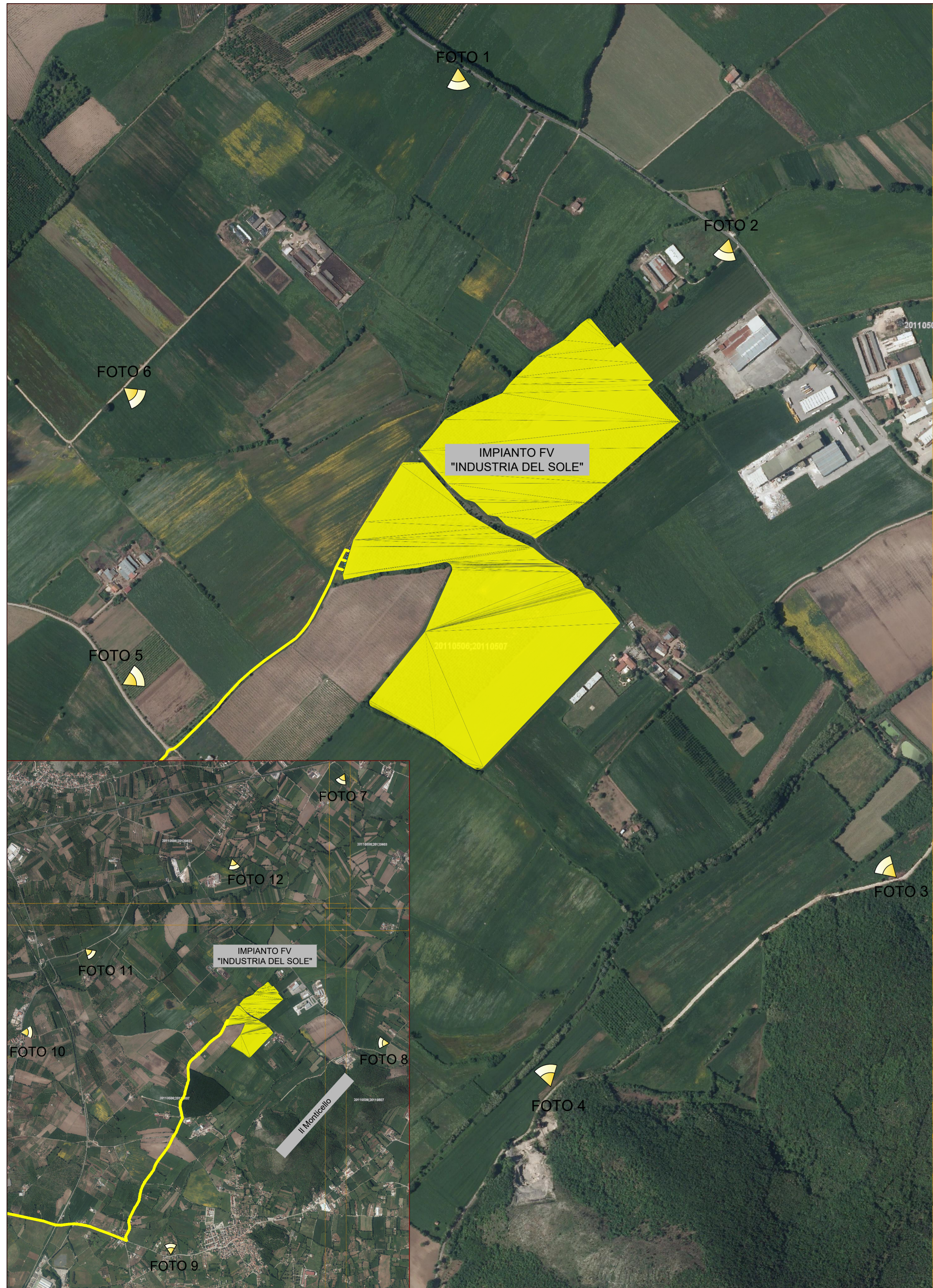
Inquadramento area impianto con coni visivi ampio raggio scala 1:30.000 Inquadramento Area impianto con coni visivi scala 1:5.000
