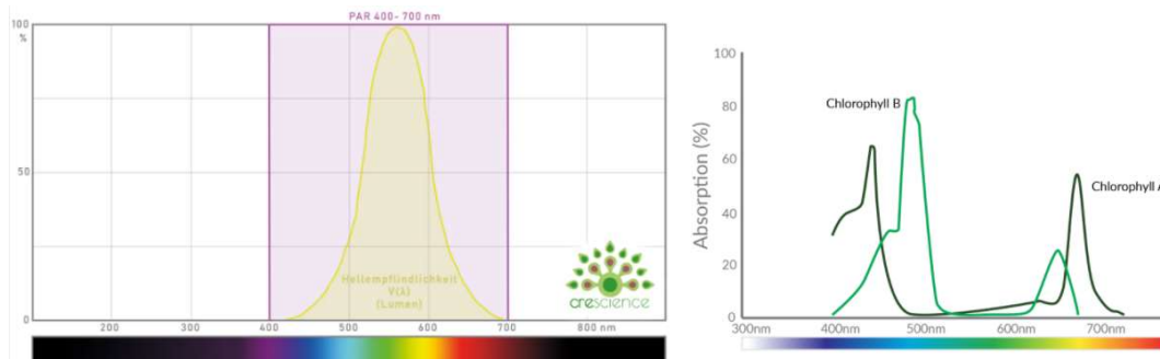
20 – la fotosintesi e la correlazione con la lunghezza d'onda
