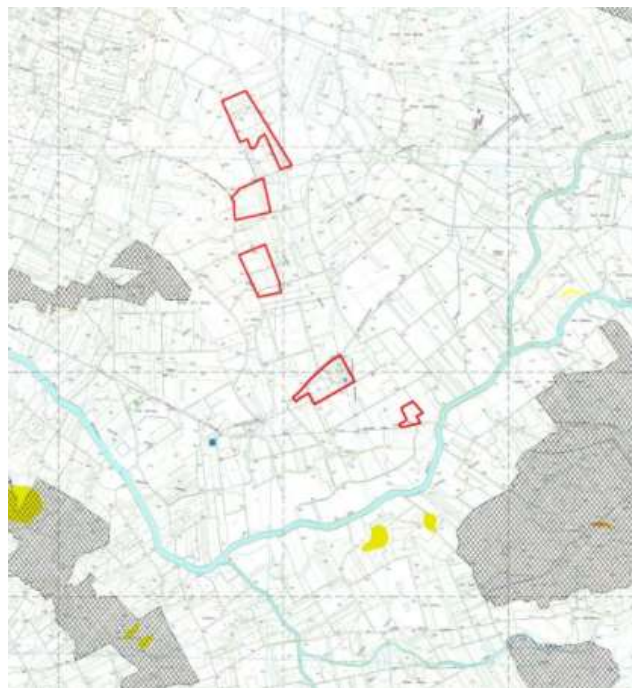
3 – Inquadramento aree di progetto su CTR 1:10000
