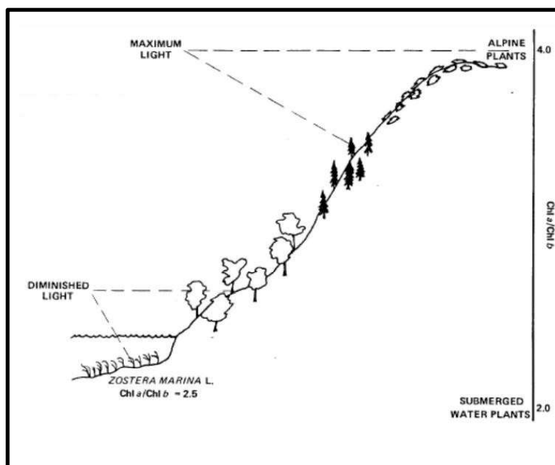
22 – gli effetti della luce in funzione dell'altimetria
