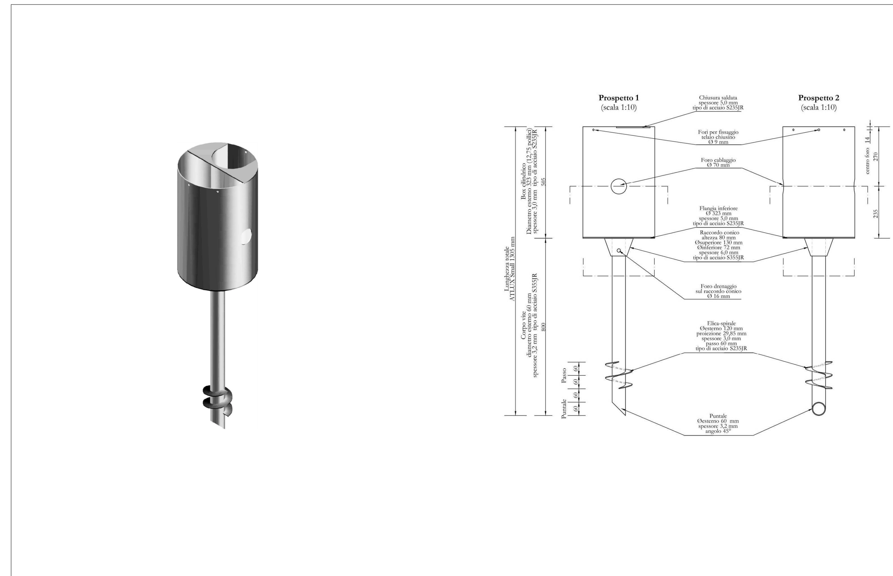
FONDAZIONE A VITE PER PALI DI FONDAZIONE del tipo 'ATLANTECH'
