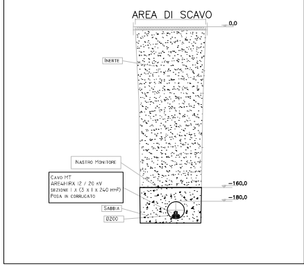
PARTICOLARE SEZIONE SCAVO SINGOLO CAVIDOTTO
