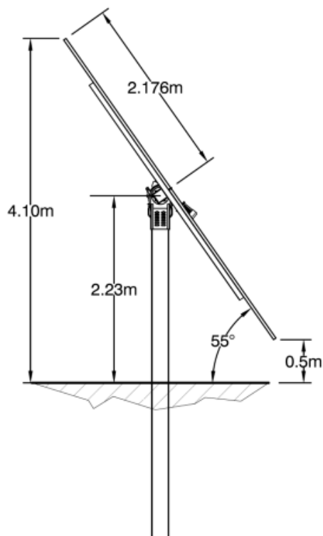
Particolare struttura di supporto
