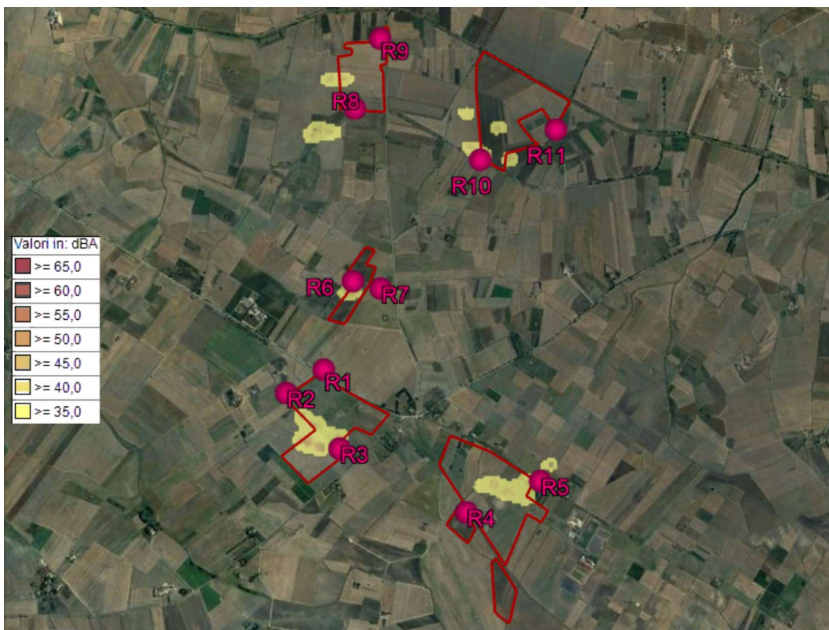
Fig. 7.1 – Mappa isofoniche da simulazione con MMS Nftplso9613
